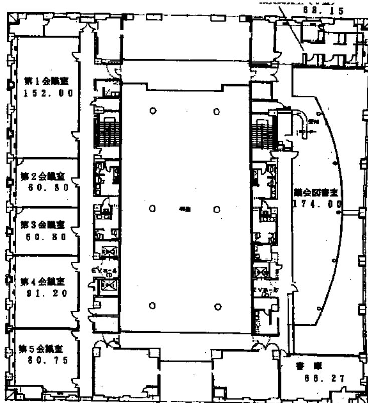
2階平面図
