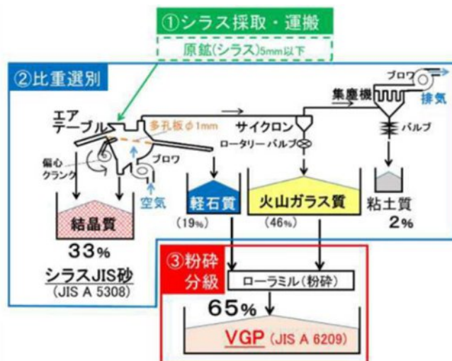
VGP の製造工程
