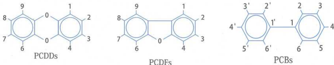
図3-34 ダイオキシン類の構造式
