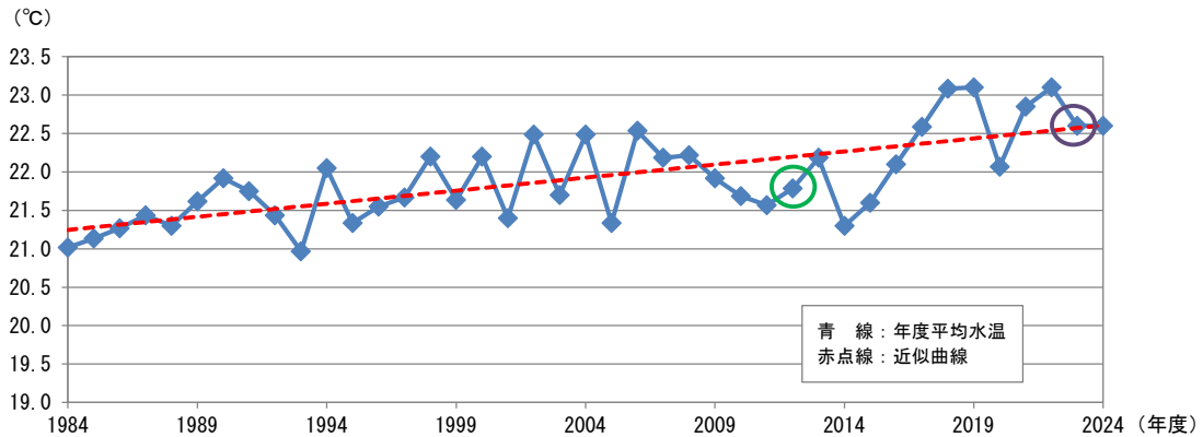
図 1-13 鹿児島湾の年度平均水温の経年変化
