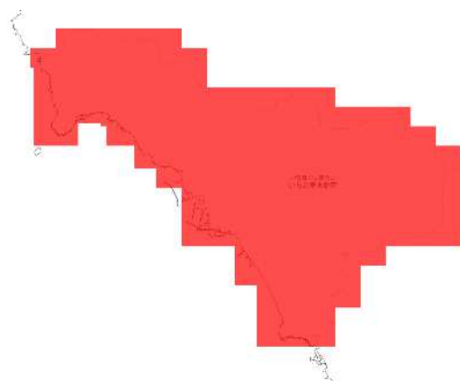
RCP 8.5 2091-2100年
