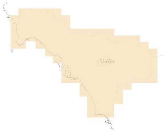
RCP 2.6 2091-2100年
