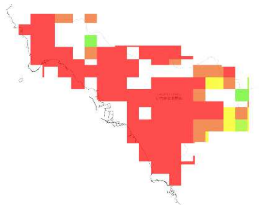
RCP 8.5 21世紀末 出穂後20日間の日平均気温26℃以上の積算値
