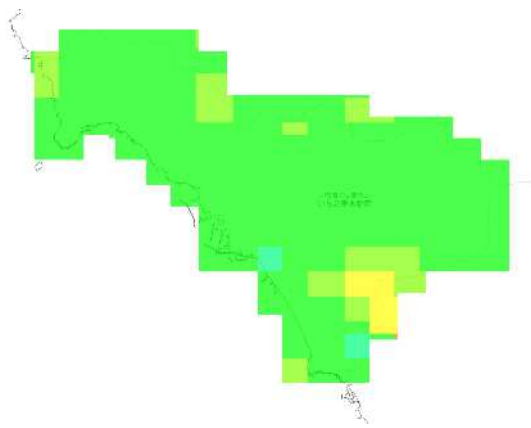
RCP 2.6 2011-2020年
