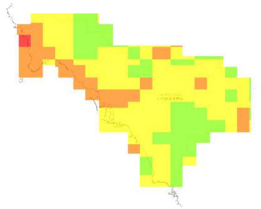
RCP 8.5 2091-2100年
