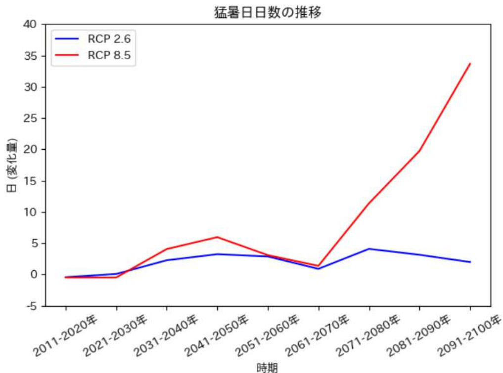
猛暑日の推移予測 (いちき串木野市)
