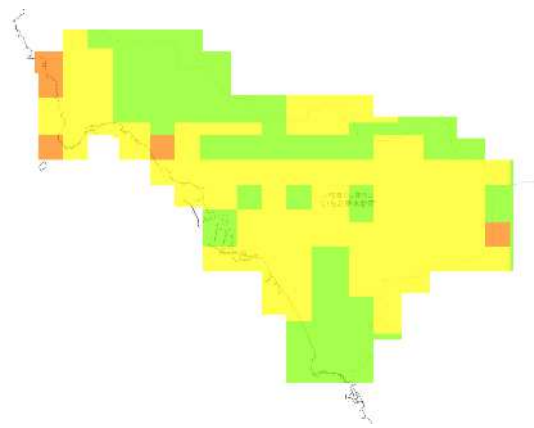
RCP 8.5 2011-2020年
