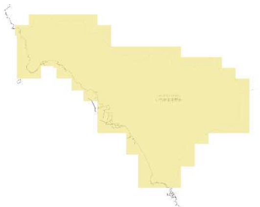
RCP 2.6 2091-2100年
