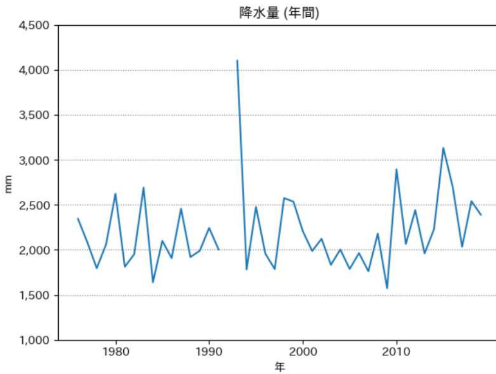
年間降水量の推移 (東市来)
