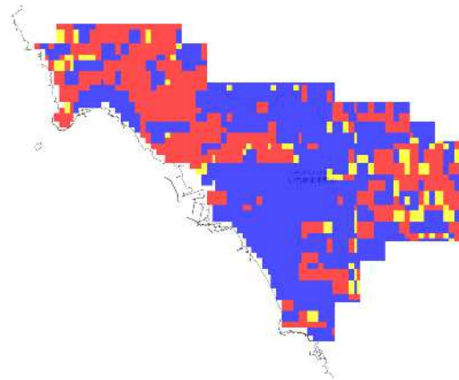
RCP 8.5 2081-2100年
