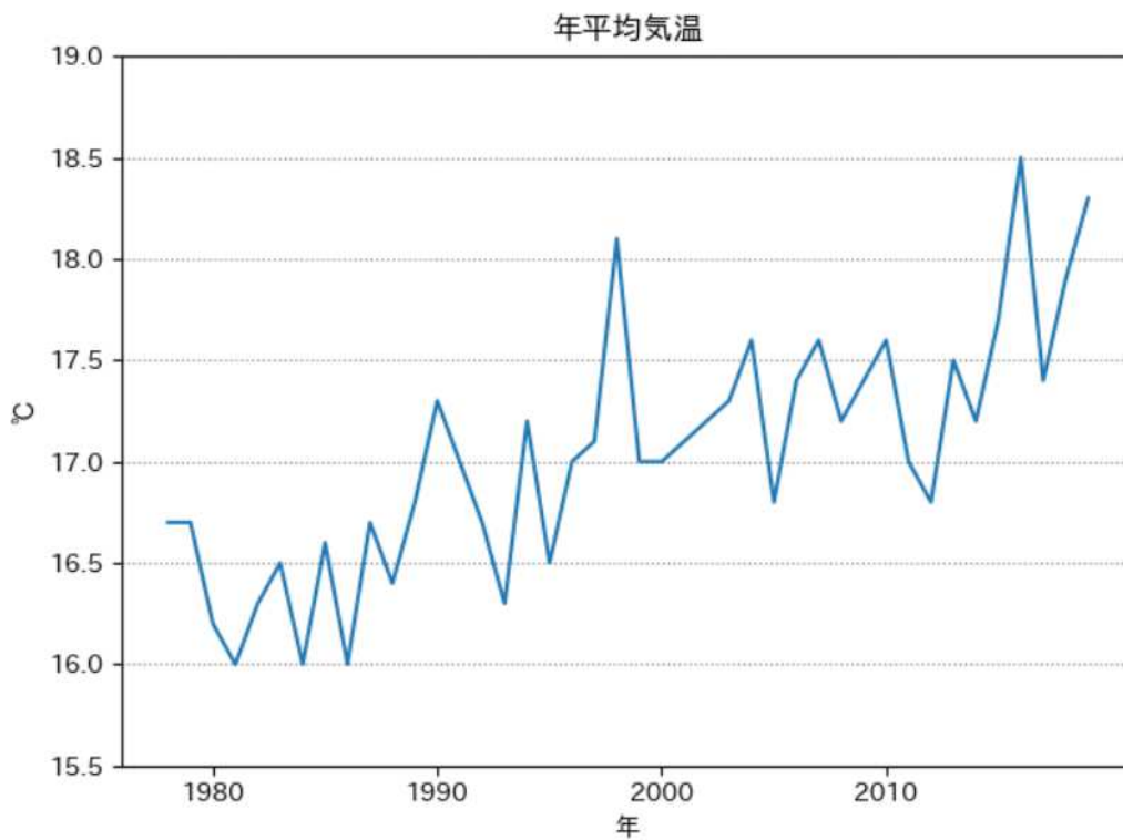
年平均気温の推移 (東市来)
