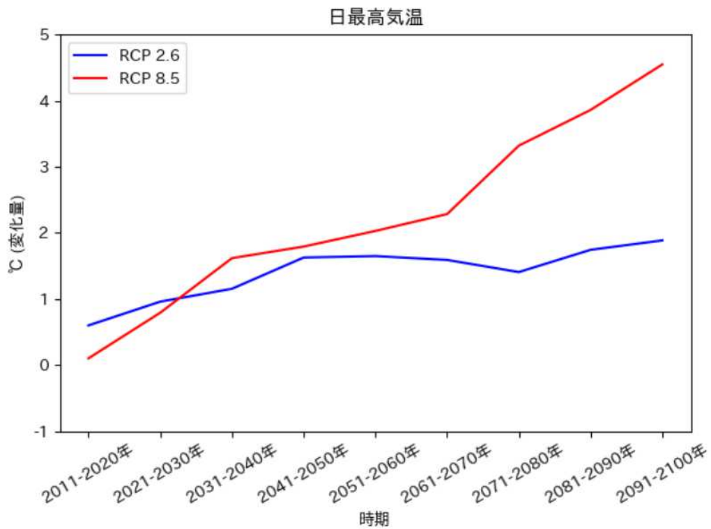
日最高気温の推移予測 (いちき串木野市)
