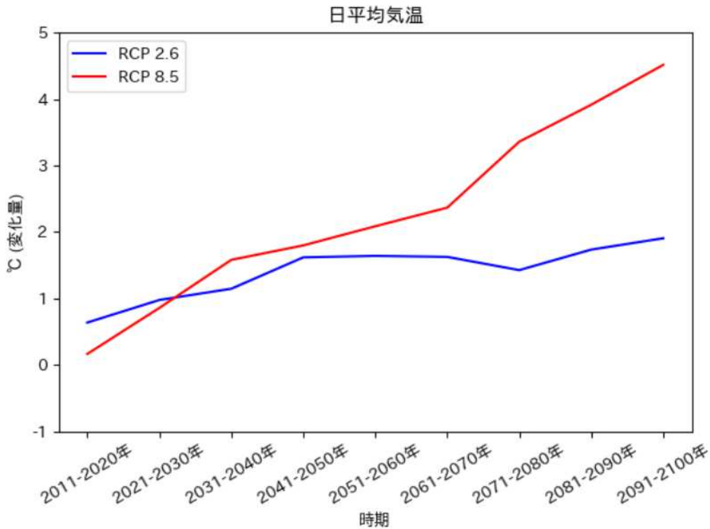
日平均気温の推移予測 (いちき串木野市)
