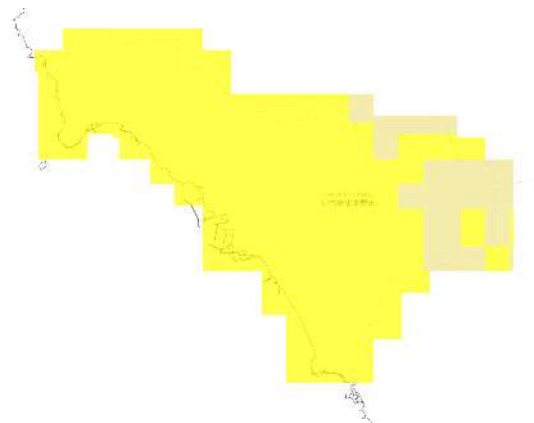
RCP 8.5 2051-2060年
