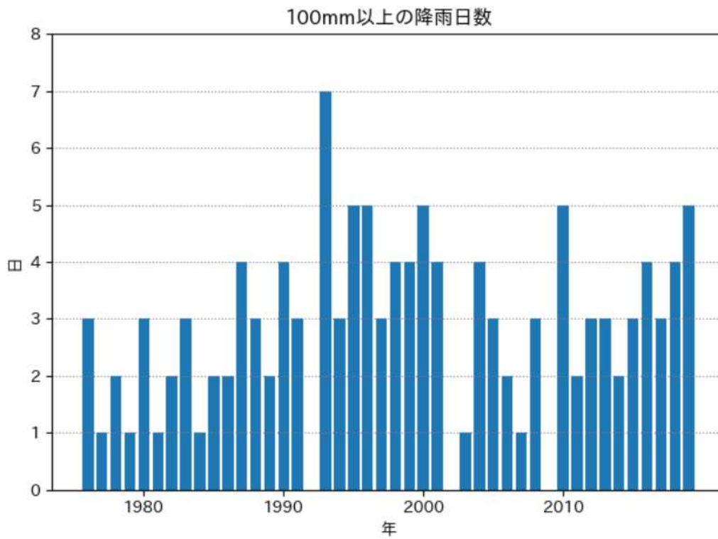
100mm以上の降雨日数の推移（東市来）
