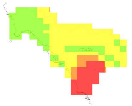
RCP 8.5 2051-2060年
