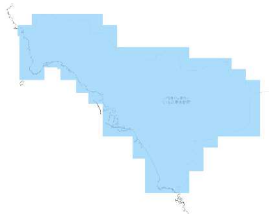
RCP 8.5 2091-2100年
