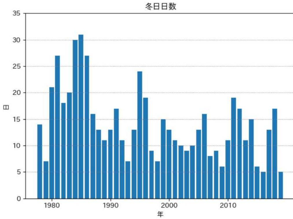
冬日日数の推移 (東市来)
