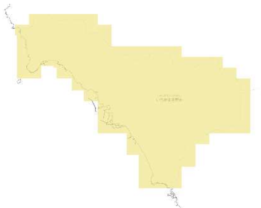
RCP 2.6 2051-2060年
