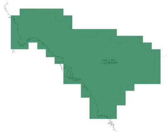
RCP 8.5 21世紀半ば
