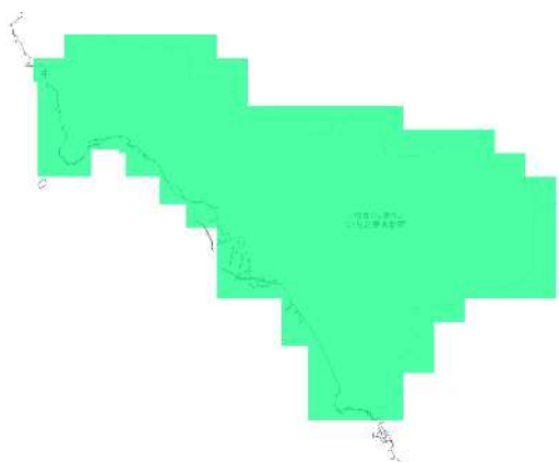
RCP 2.6 2091-2100年
