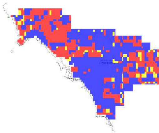
RCP 2.6 2081-2100年
