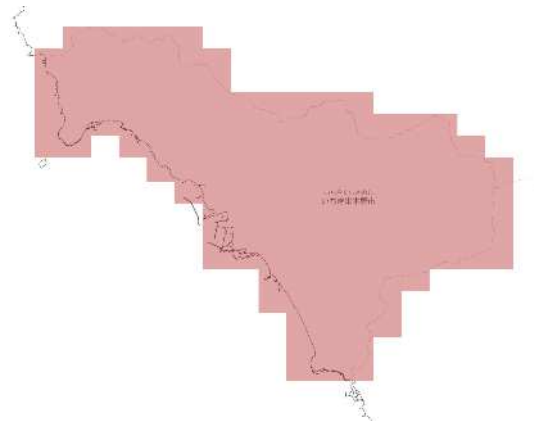
RCP 8.5 21世紀末
