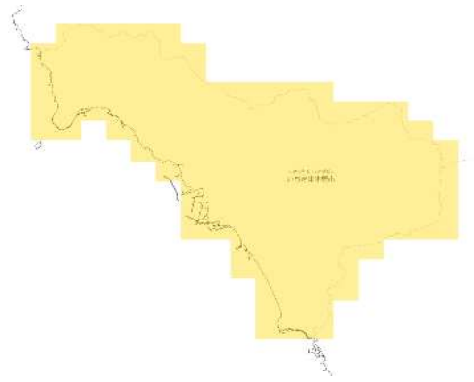
RCP 8.5 21世紀末
