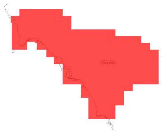
RCP 8.5 2091-2100年
