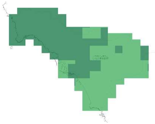
RCP 2.6 21世紀末
