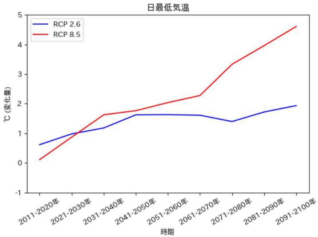
日最低気温の推移予測 (いちき串木野市)
