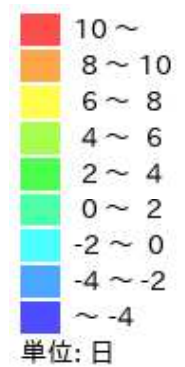
RCP 8.5 2091-2100年
