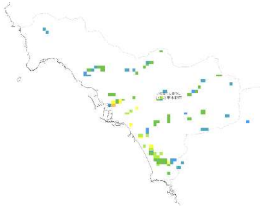
RCP 2.6 2081-2100年
