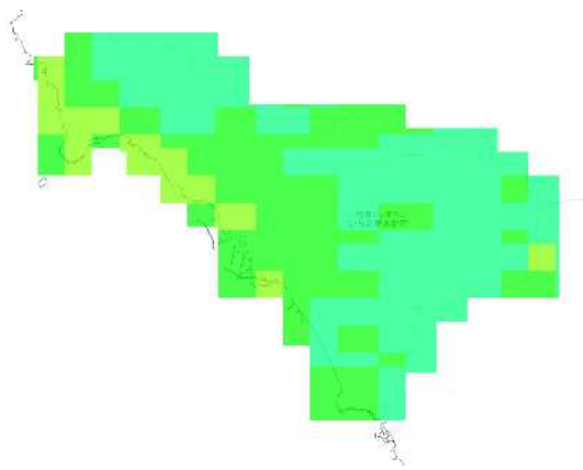
RCP 2.6 2051-2060年
