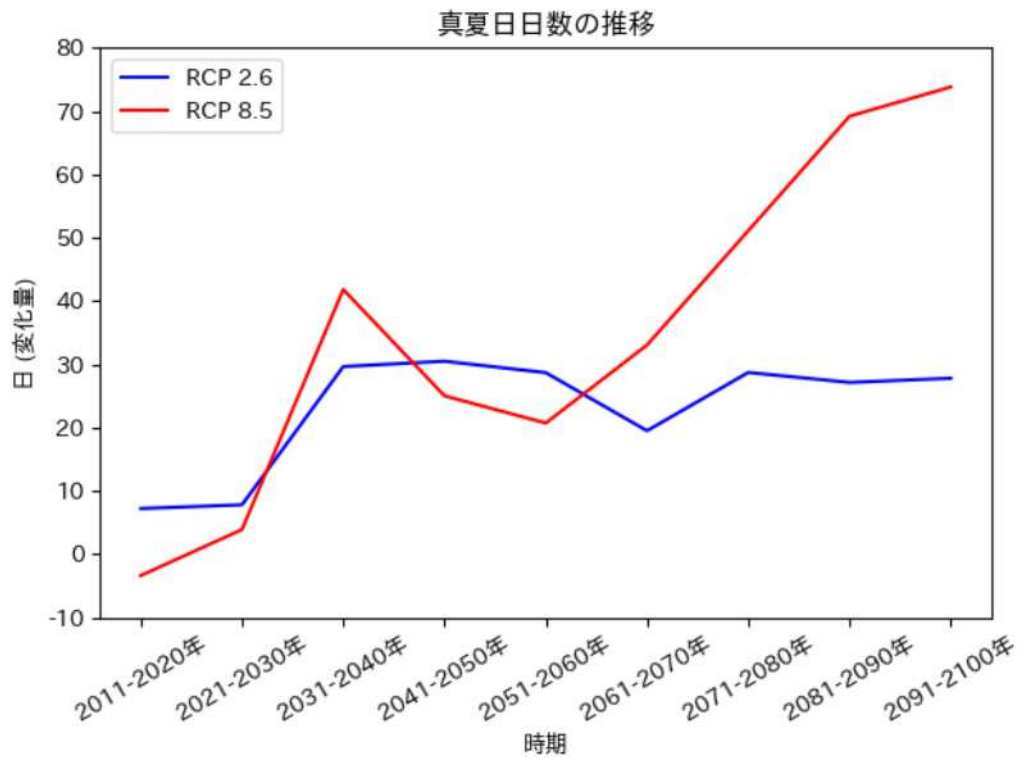
真夏日の推移予測 (いちき串木野市)
