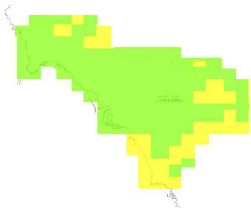
RCP 2.6 2051-2060年
