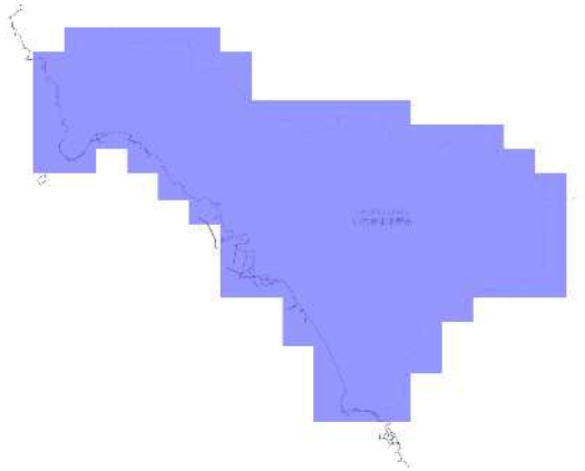
RCP 2.6 21世紀末
