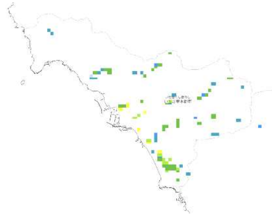
RCP 8.5 2081-2100年
