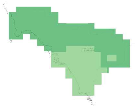
RCP 8.5 21世紀末
