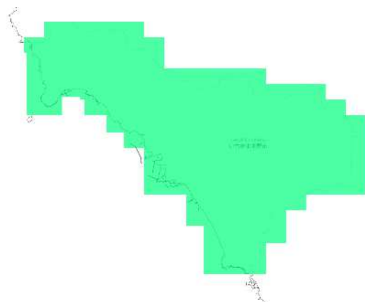
RCP 8.5 2051-2060年
