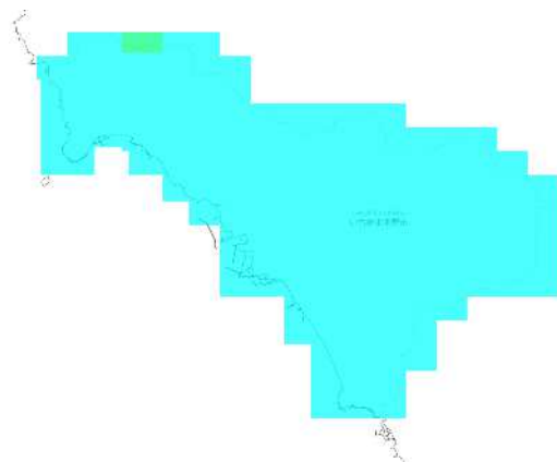
RCP 8.5 2011-2020年
