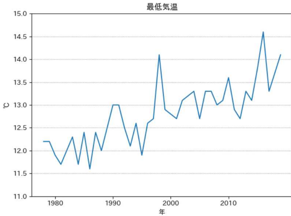
日最低気温の年平均の推移 (東市来)
