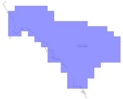
RCP 8.5 21世紀末
