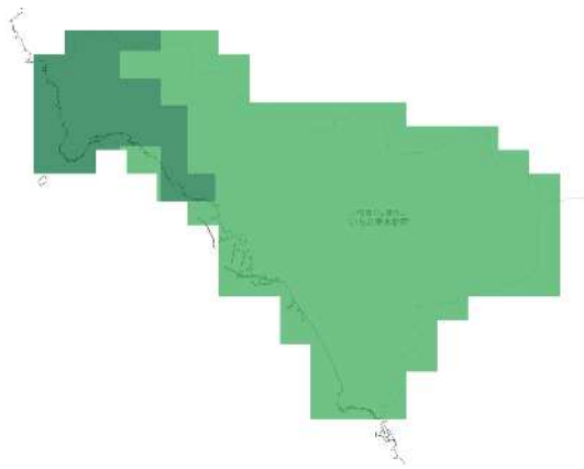
RCP 2.6 21世紀半ば
