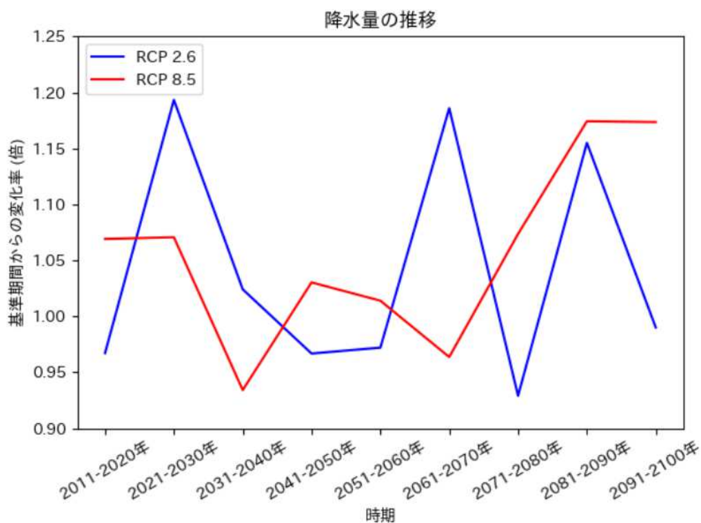
降水量の推移予測 (いちき串木野市)
