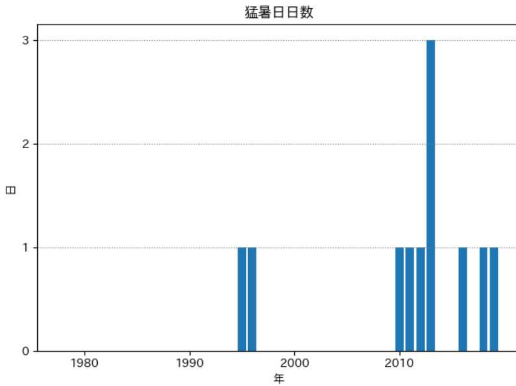
猛暑日日数の推移（東市来）
