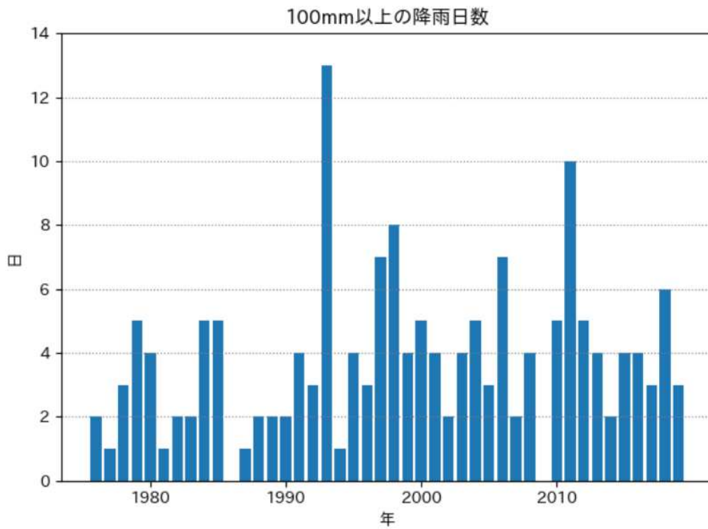
100mm以上の降雨日数の推移（大口）
