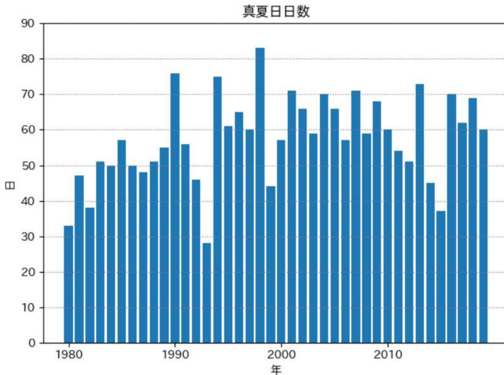
真夏日日数の推移 (大口)
