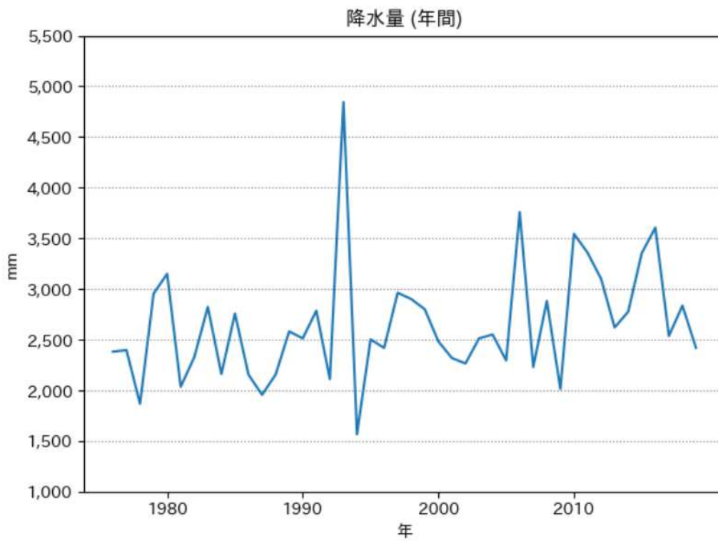
間降水量の推移 (大口)
