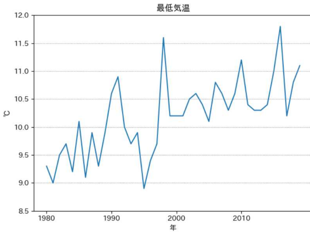
日最低気温の年平均の推移 (大口)
