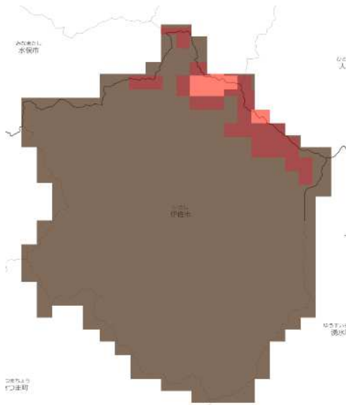
RCP 2.6 21世紀半ば
