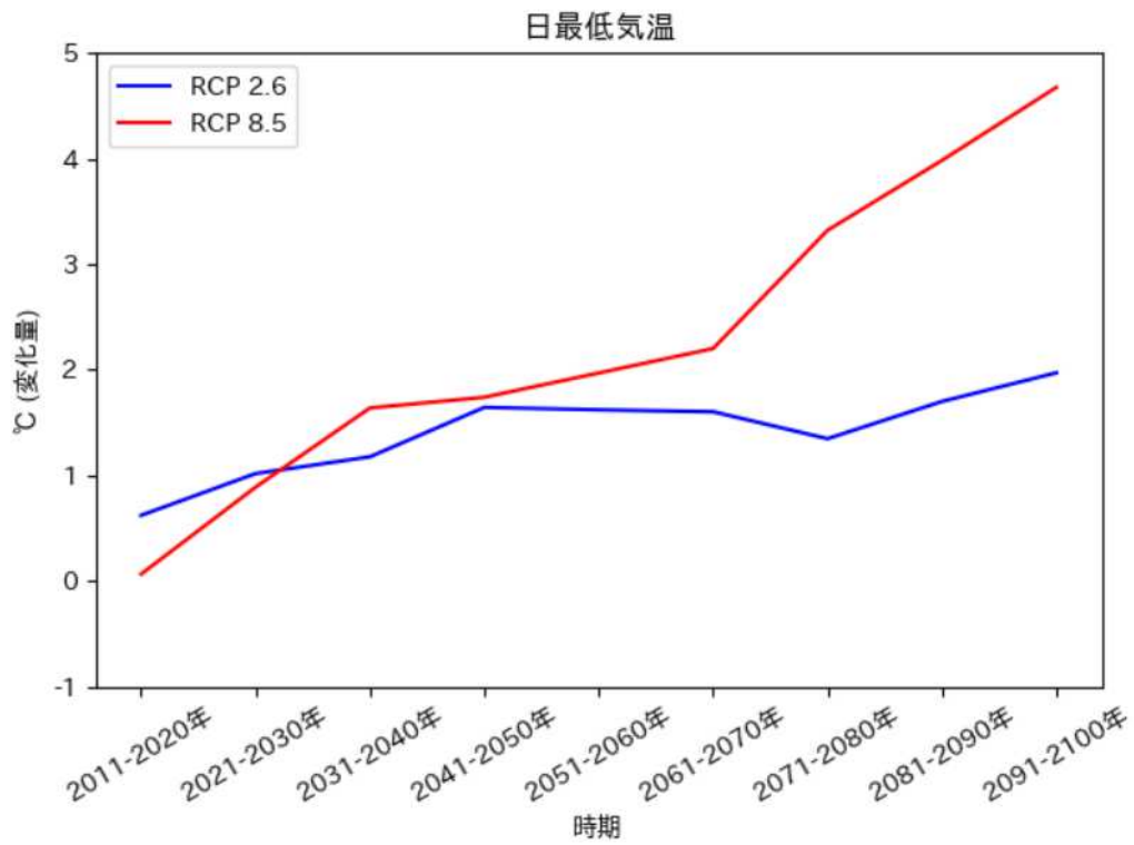
日最低気温の推移予測 (伊佐市)
