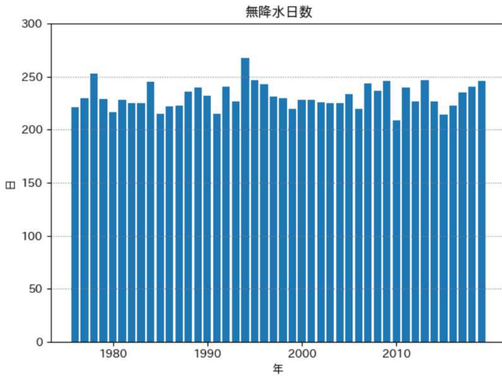
年間無降水日数の推移（大口）
