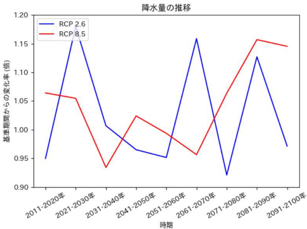
降水量の推移予測 (伊佐市)
