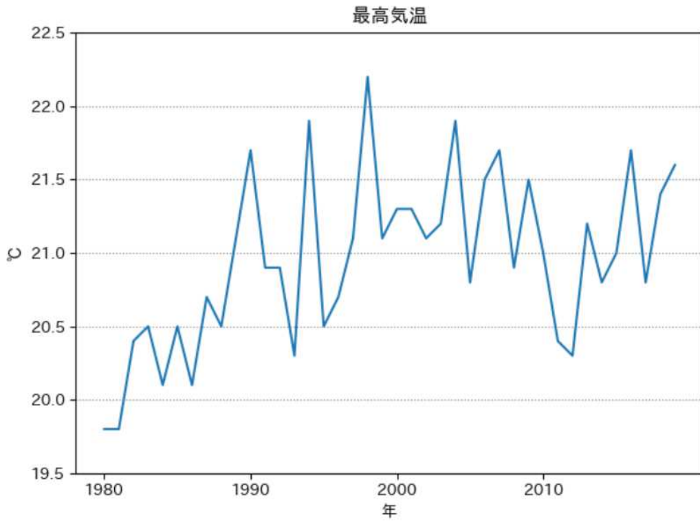
日最高気温の年平均の推移 (大口)
