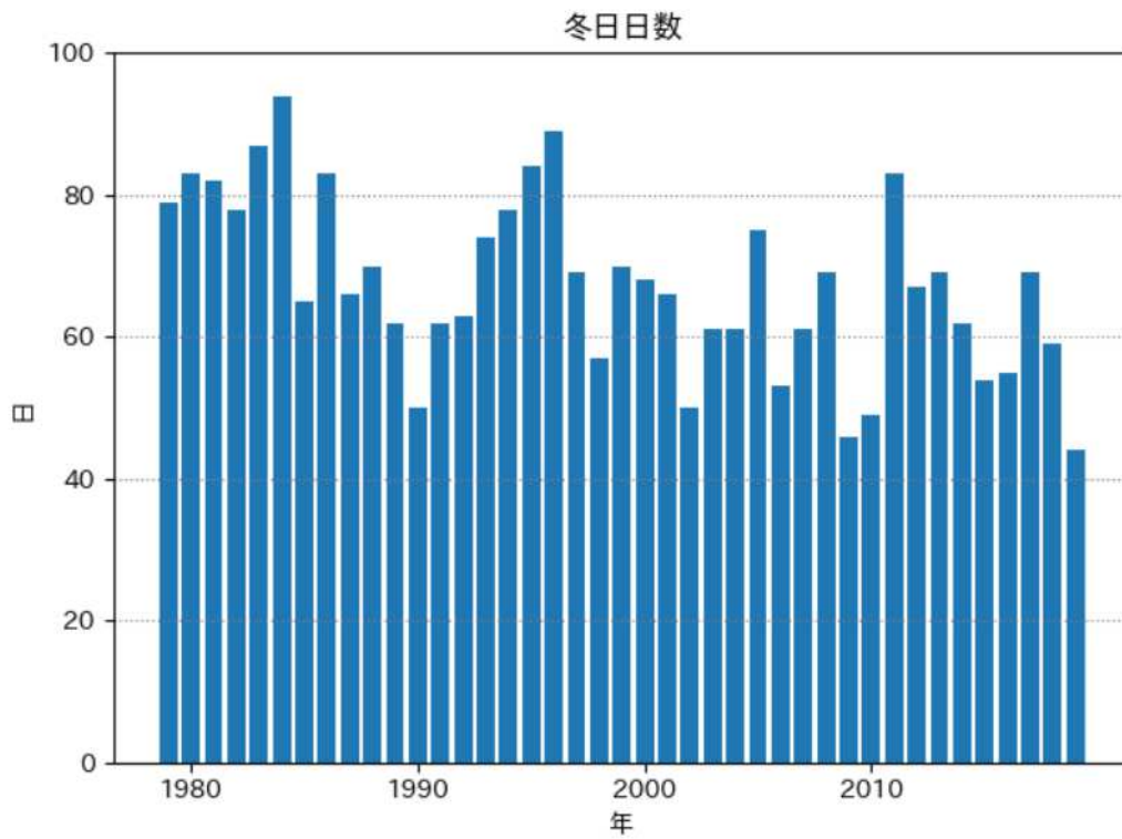
冬日日数の推移 (大口)
