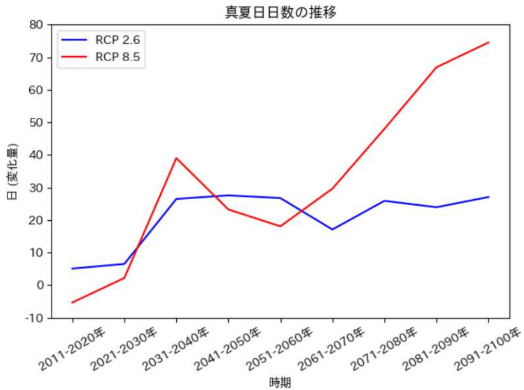
真夏日の推移予測（伊佐市）
