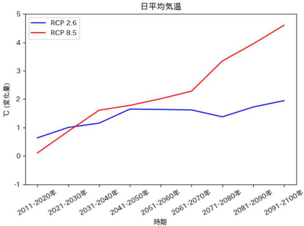
日平均気温の推移予測 (伊佐市)
