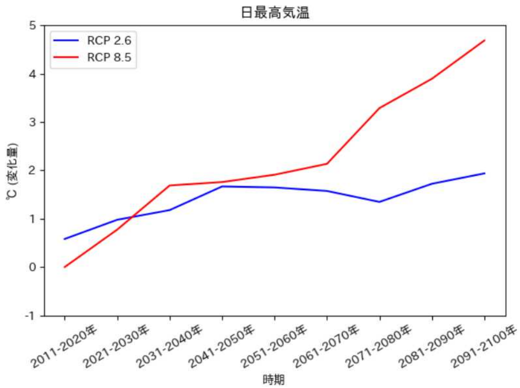
日最高気温の推移予測 (伊佐市)
