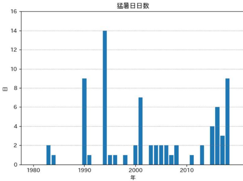
猛暑日日数の推移（大口）
