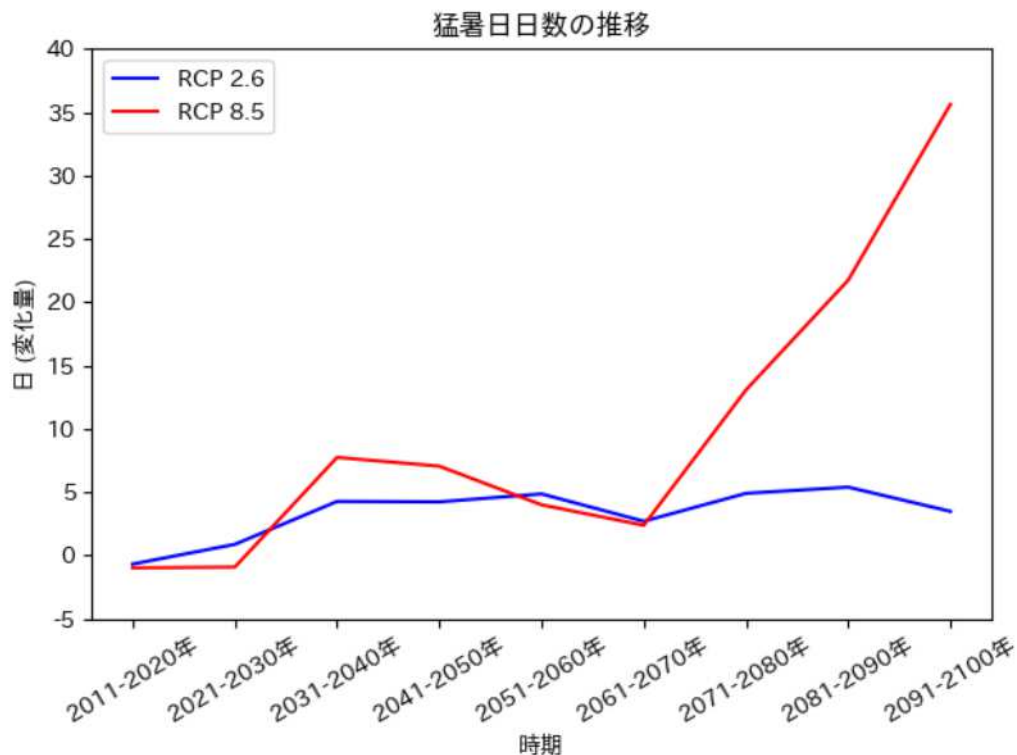
図 27 猛暑日の推移予測 (伊佐市)
