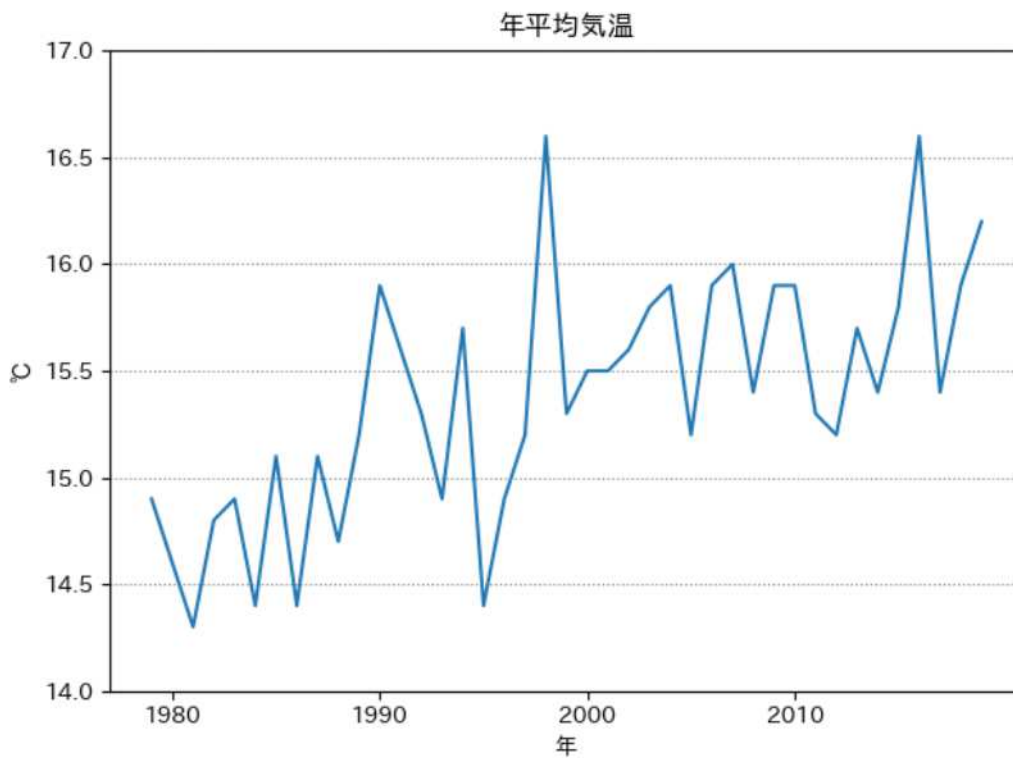
年平均気温の推移 (大口)
