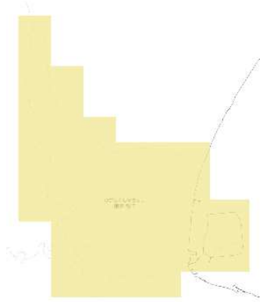
RCP 2.6 2051-2060年
