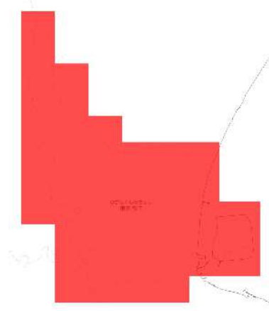
RCP 8.5 2091-2100年
