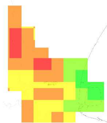
RCP 8.5 2091-2100年
