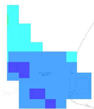
RCP 8.5 2051-2060年
