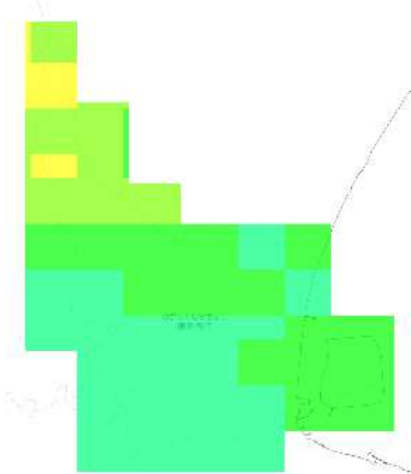
RCP 2.6 2091-2100年
