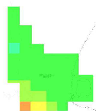
RCP 8.5 2011-2020年
