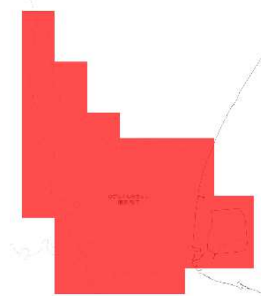
RCP 8.5 2091-2100年
