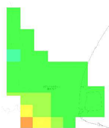
RCP 2.6 2011-2020年
