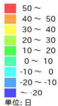
RCP 8.5 2091-2100年
