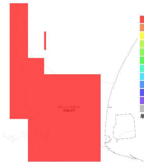
RCP 2.6 21世紀末
