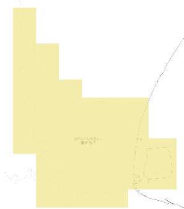
RCP 2.6 2091-2100年
