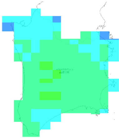
RCP 2.6 2011-2020年
