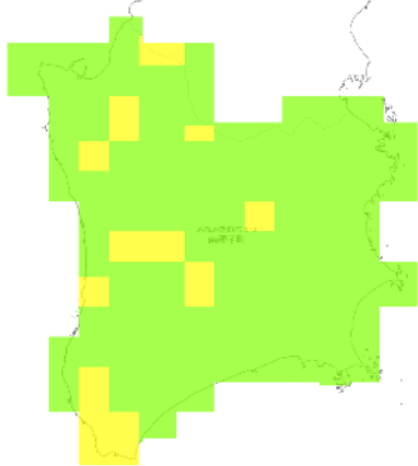
RCP 2.6 2051-2060年
