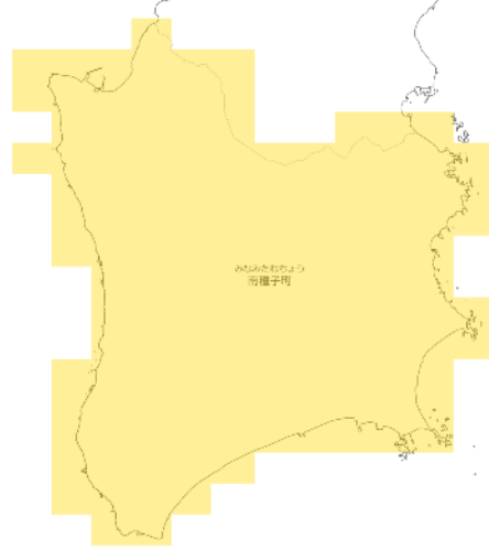
RCP 8.5 21世紀末
