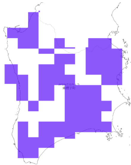
RCP 8.5 21世紀末
