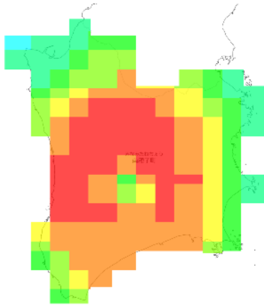
RCP 2.6 2011-2020年
