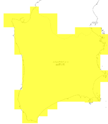
RCP 8.5 2051-2060年
