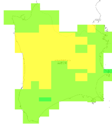
RCP 8.5 2091-2100年
