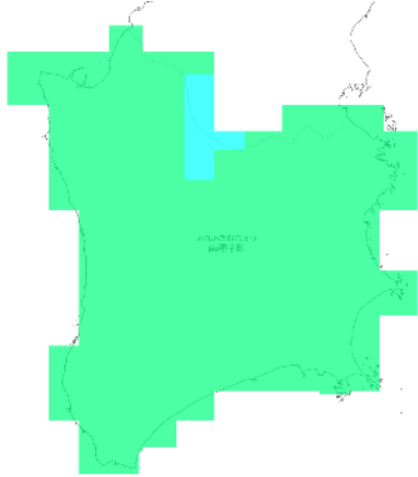
RCP 2.6 2051-2060年
