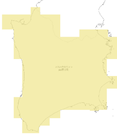
RCP 2.6 2051-2060年
