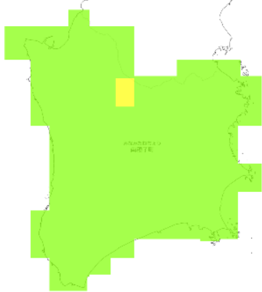
RCP 2.6 2091-2100年
