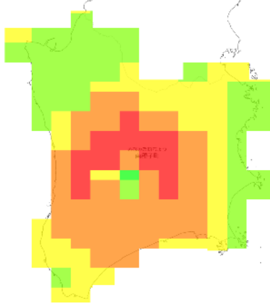
RCP 2.6 2051-2060年
