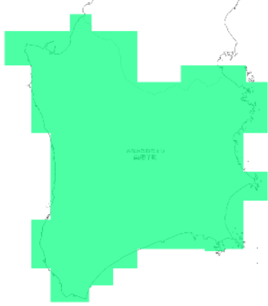
RCP 2.6 2091-2100年
