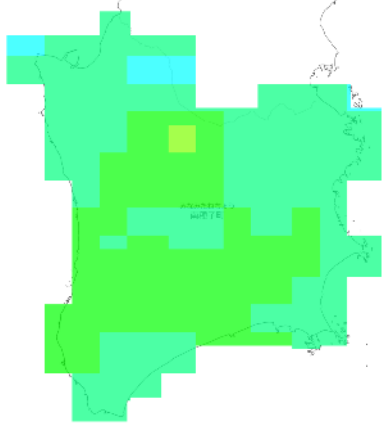
RCP 2.6 2091-2100年
