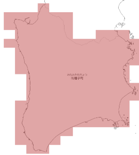
RCP 8.5 21世紀末
