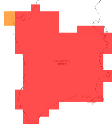
RCP 8.5 2051-2060年
