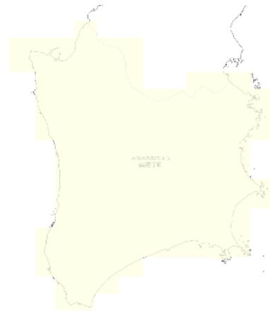
RCP 8.5 2011-2020年
