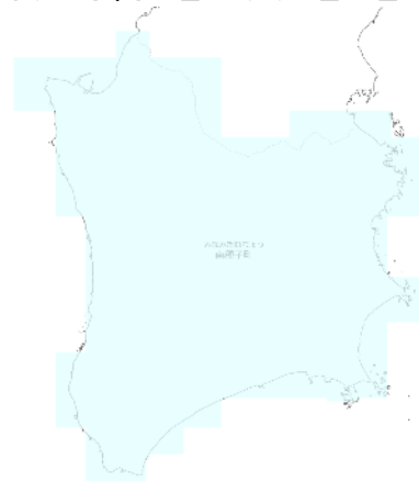
RCP 8.5 2051-2060年
