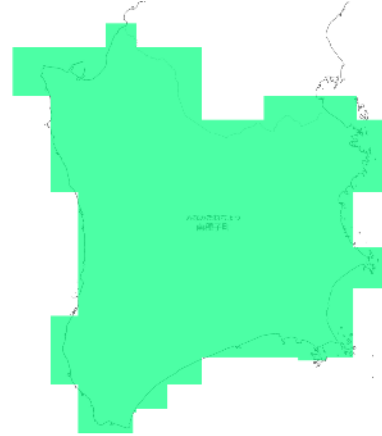
RCP 8.5 2051-2060年
