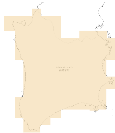
RCP 8.5 2011-2020年
