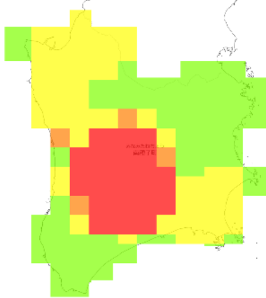
RCP 2.6 2091-2100年
