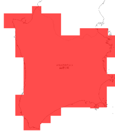
RCP 8.5 2091-2100年
