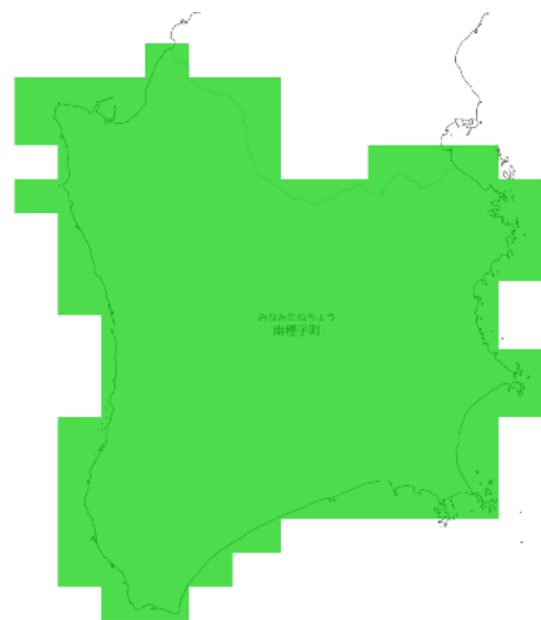
RCP 8.5 21世紀末
