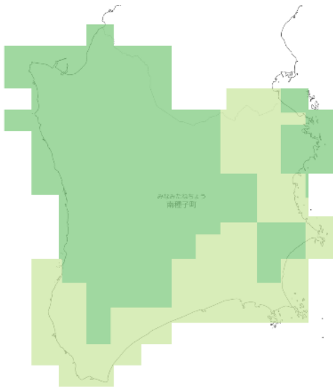
RCP 2.6 21世紀末
