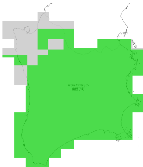
RCP 2.6 21世紀末
