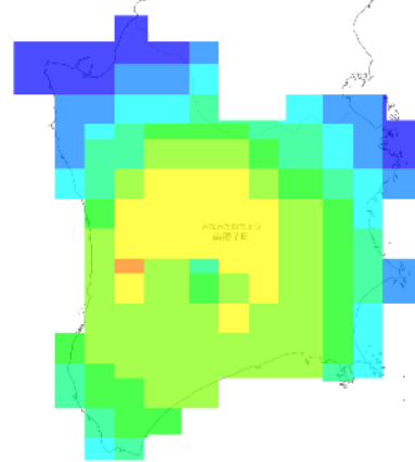
RCP 8.5 2091-2100年
