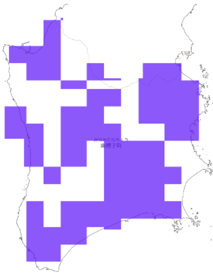
RCP 2.6 21世紀末
