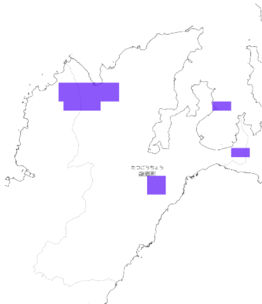
RCP 2.6 21世紀末
