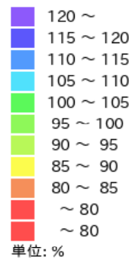
RCP 8.5 21世紀末
