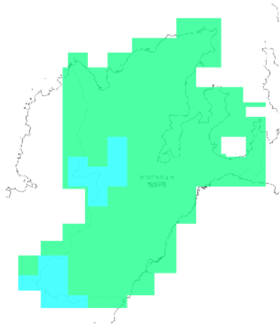
RCP 2.6 2051-2060年
