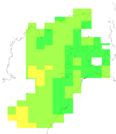
RCP 2.6 2051-2060年
