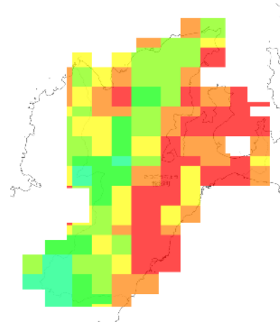
RCP 8.5 2091-2100年
