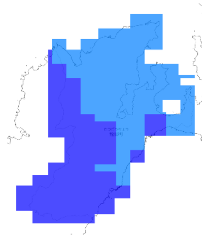
RCP 8.5 2011-2020年
