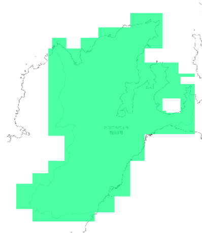
RCP 8.5 2051-2060年
