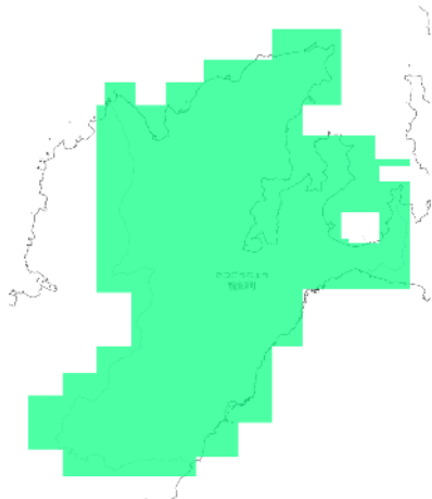
RCP 2.6 2011-2020年
