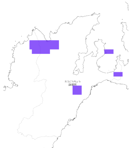
RCP 8.5 21世紀末
