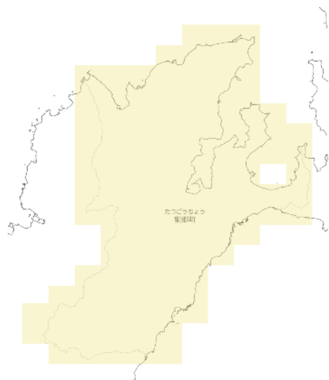
RCP 2.6 21世紀末
