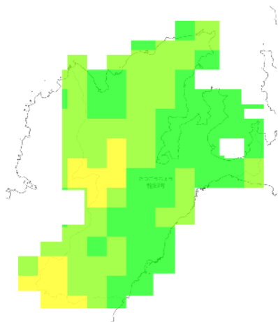
RCP 2.6 2091-2100年
