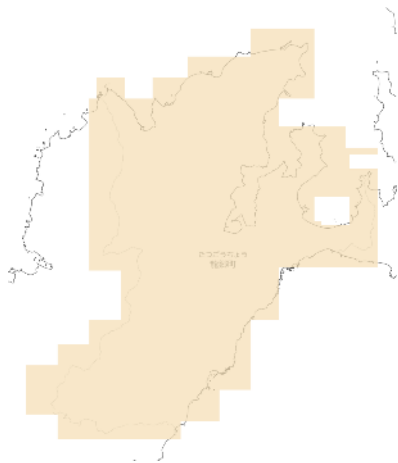
RCP 2.6 2091-2100年
