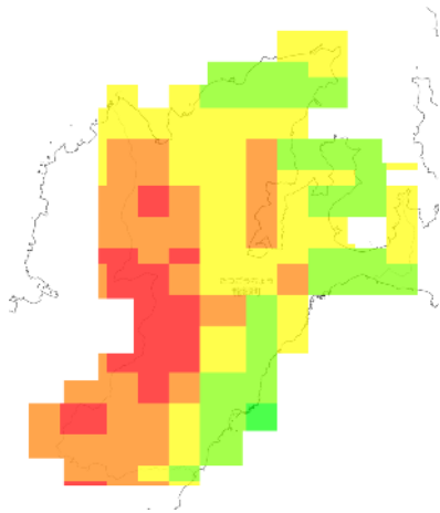
RCP 2.6 2011-2020年
