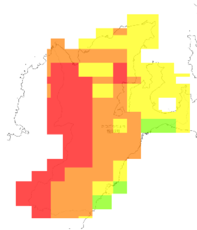
RCP 8.5 2091-2100年
