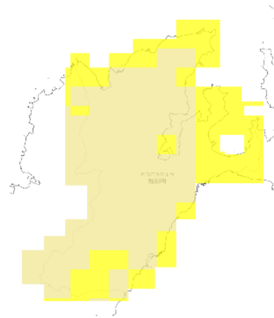
RCP 8.5 2051-2060年
