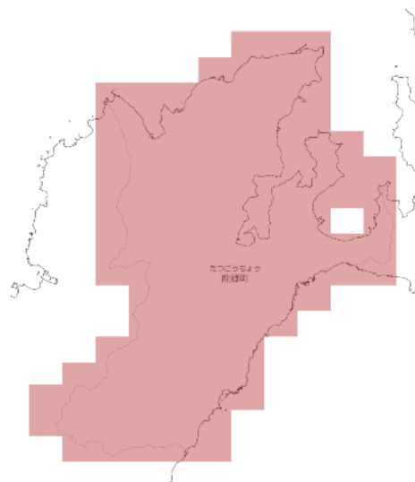
RCP 8.5 21世紀末
