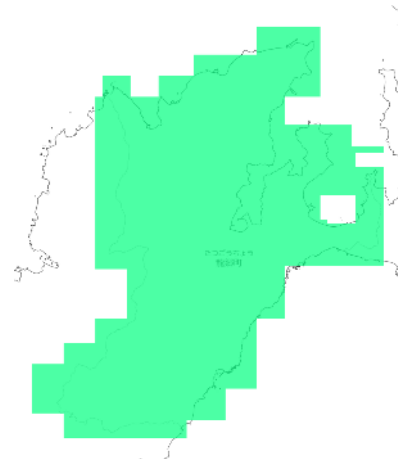
RCP 8.5 2011-2020年
