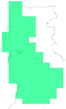
RCP 2.6 2011-2020年
