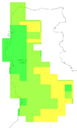
RCP 2.6 2051-2060年
