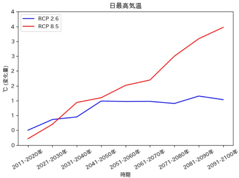
日最高気温の推移予測 (天城町)
