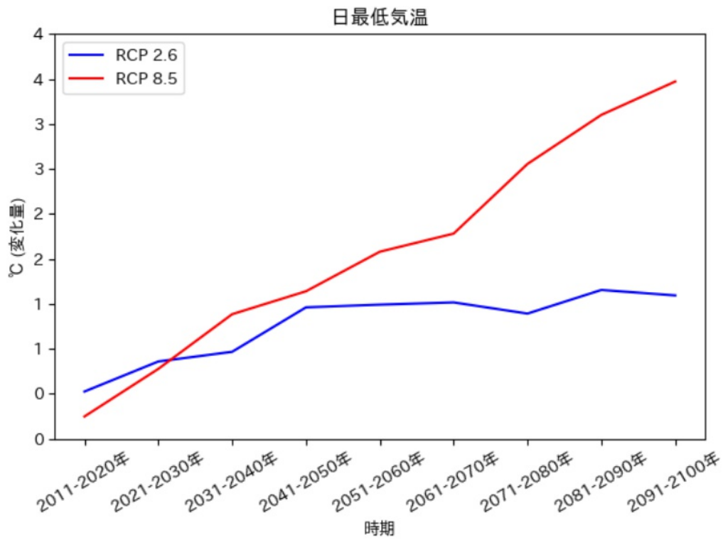
日最低気温の推移予測 (天城町)
