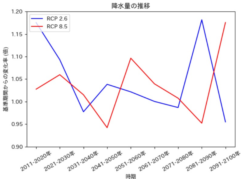
降水量の推移予測 (天城町)
