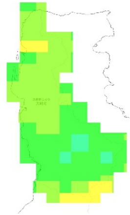
RCP 8.5 2011-2020年
