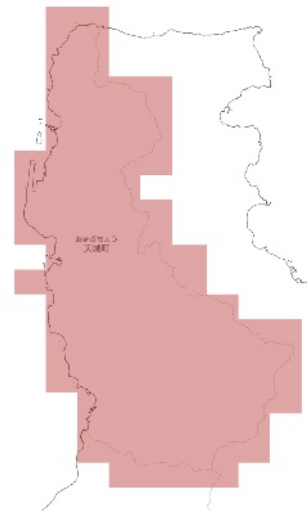
RCP 8.5 21世紀末
