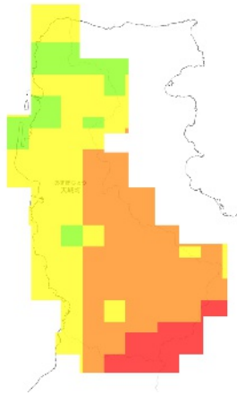
RCP 2.6 2011-2020年
