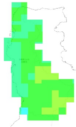
RCP 8.5 2051-2060年
