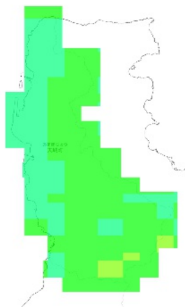
RCP 2.6 2091-2100年
