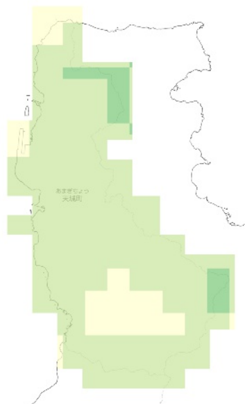
RCP 2.6 21世紀末
