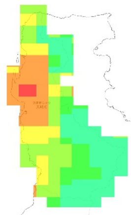
RCP 8.5 2091-2100年
