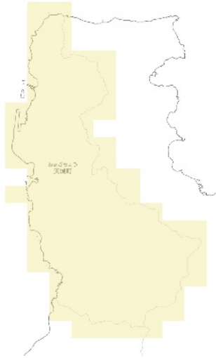
RCP 2.6 21世紀半ば
