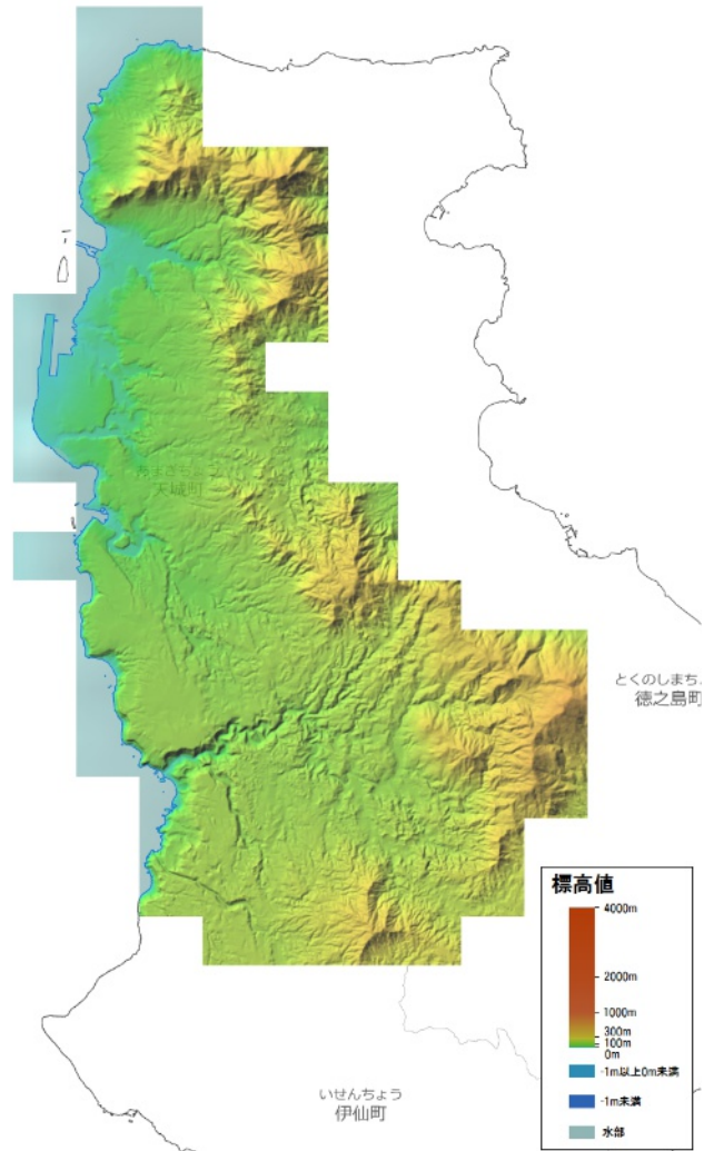
地形図 (天城町)
