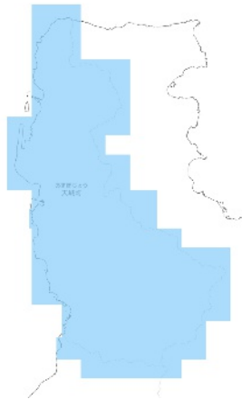
RCP 2.6 2011-2020年
