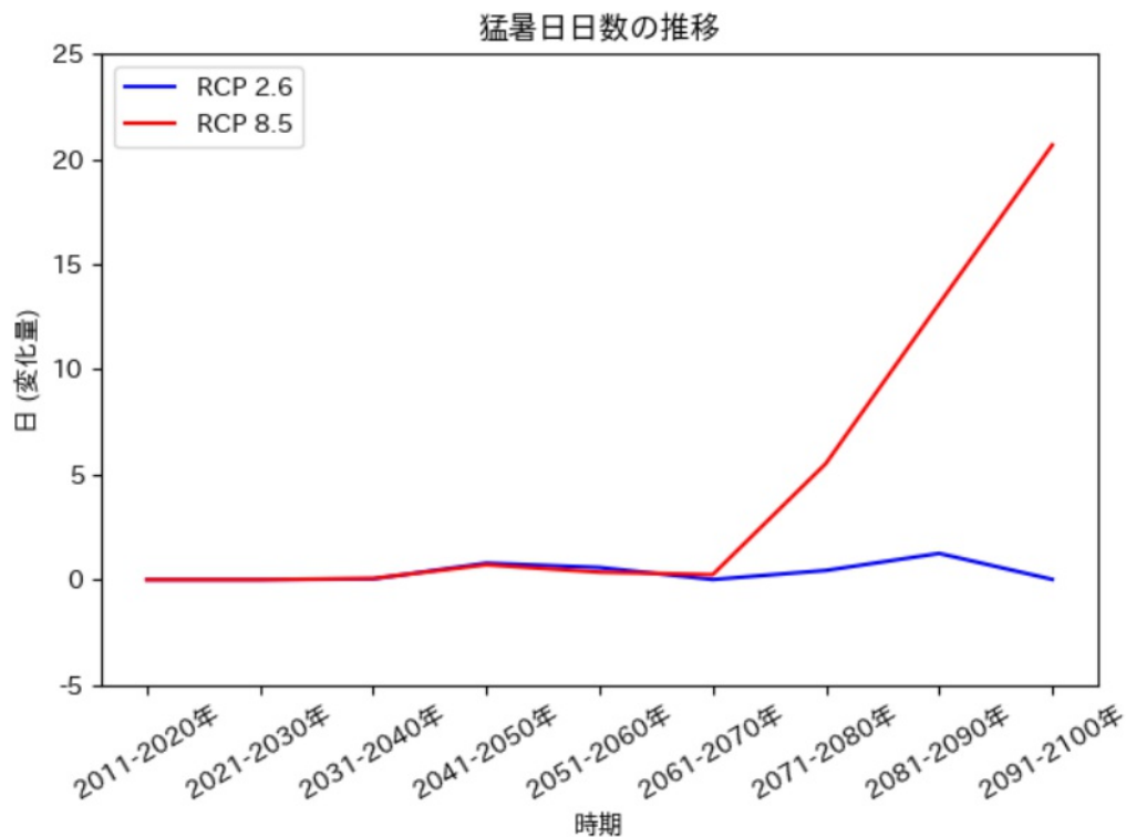
猛暑日の推移予測 (天城町)
