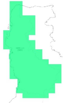
RCP 8.5 2011-2020年
