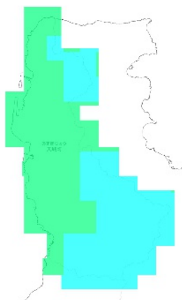
RCP 2.6 2051-2060年
