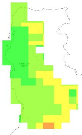
RCP 2.6 2091-2100年
