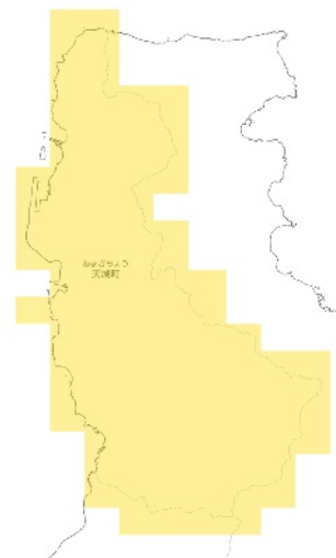
RCP 8.5 21世紀末
