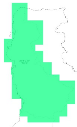
RCP 8.5 2051-2060年
