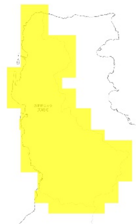
RCP 8.5 2051-2060年
