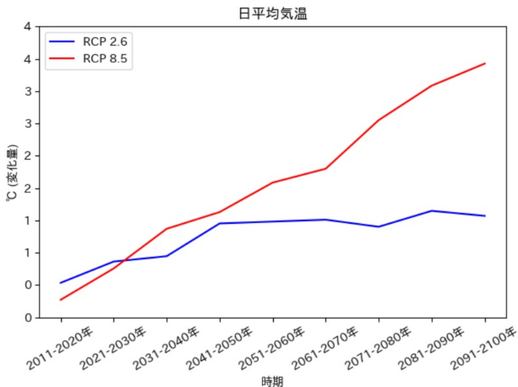
日平均気温の推移予測 (天城町)
