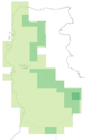
RCP 2.6 21世紀半ば
