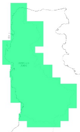
RCP 2.6 2091-2100年
