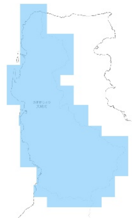
RCP 8.5 2091-2100年
