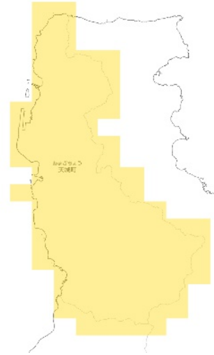
RCP 8.5 21世紀半ば
