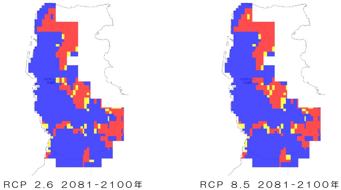
斜面崩壊発生確率
