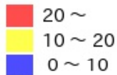
斜面崩壊発生確率 凡例
