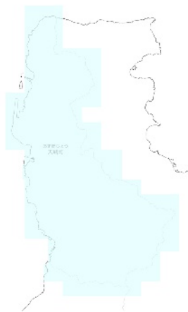
RCP 2.6 2051-2060年
