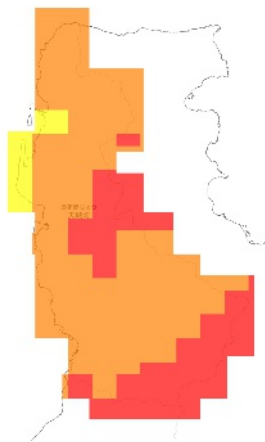
RCP 2.6 2051-2060年
