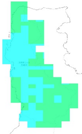
RCP 2.6 2011-2020年
