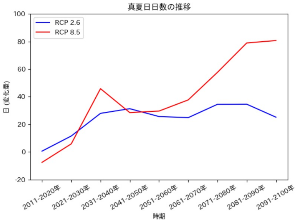
真夏日の推移予測 (天城町)
