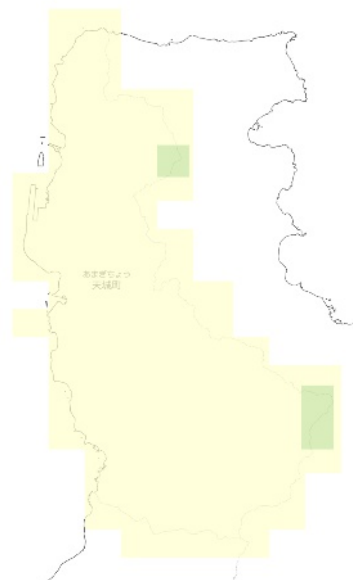
RCP 8.5 21世紀末
