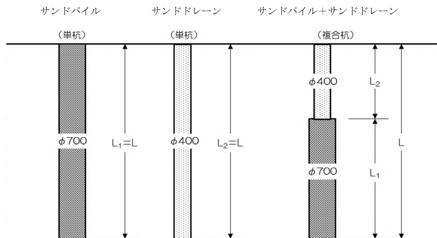
図 6-2 施工図
