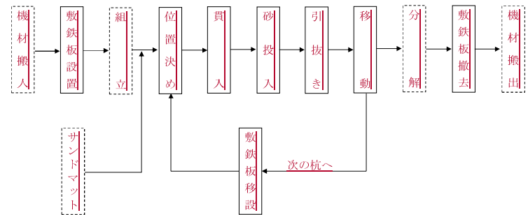
図 6－1 施工フロー
