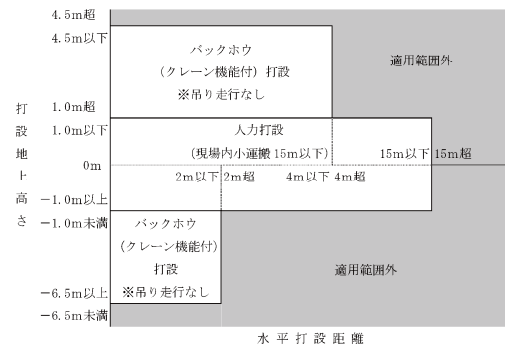
図3-1 コンクリート打設工法の選定
