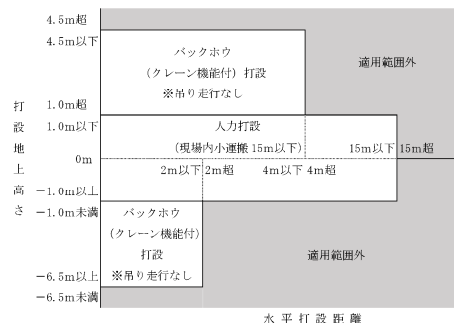
図3-1 コンクリート打設工法の選定
