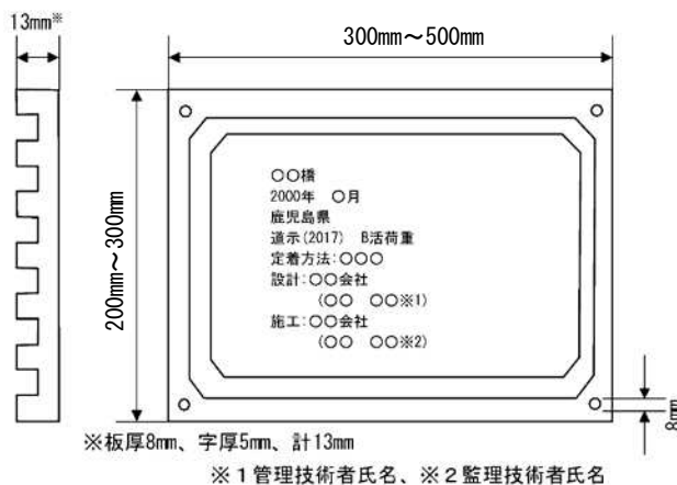
図3-2-2 銘板の寸法及び記載事項
