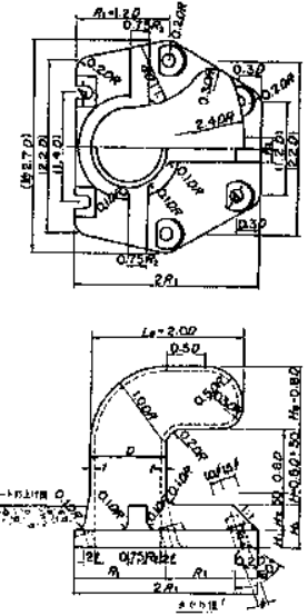
設計けん引力が350, 500, 700, 1000kNの場合
