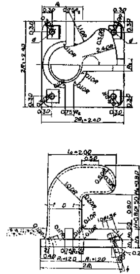
設計けん引力が50, 100, 150, 250kNの場合
