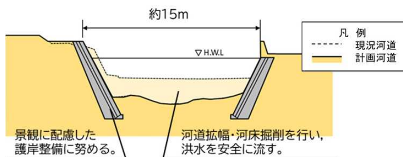
図32 稲荷川横断イメージ図（1k600付近）
