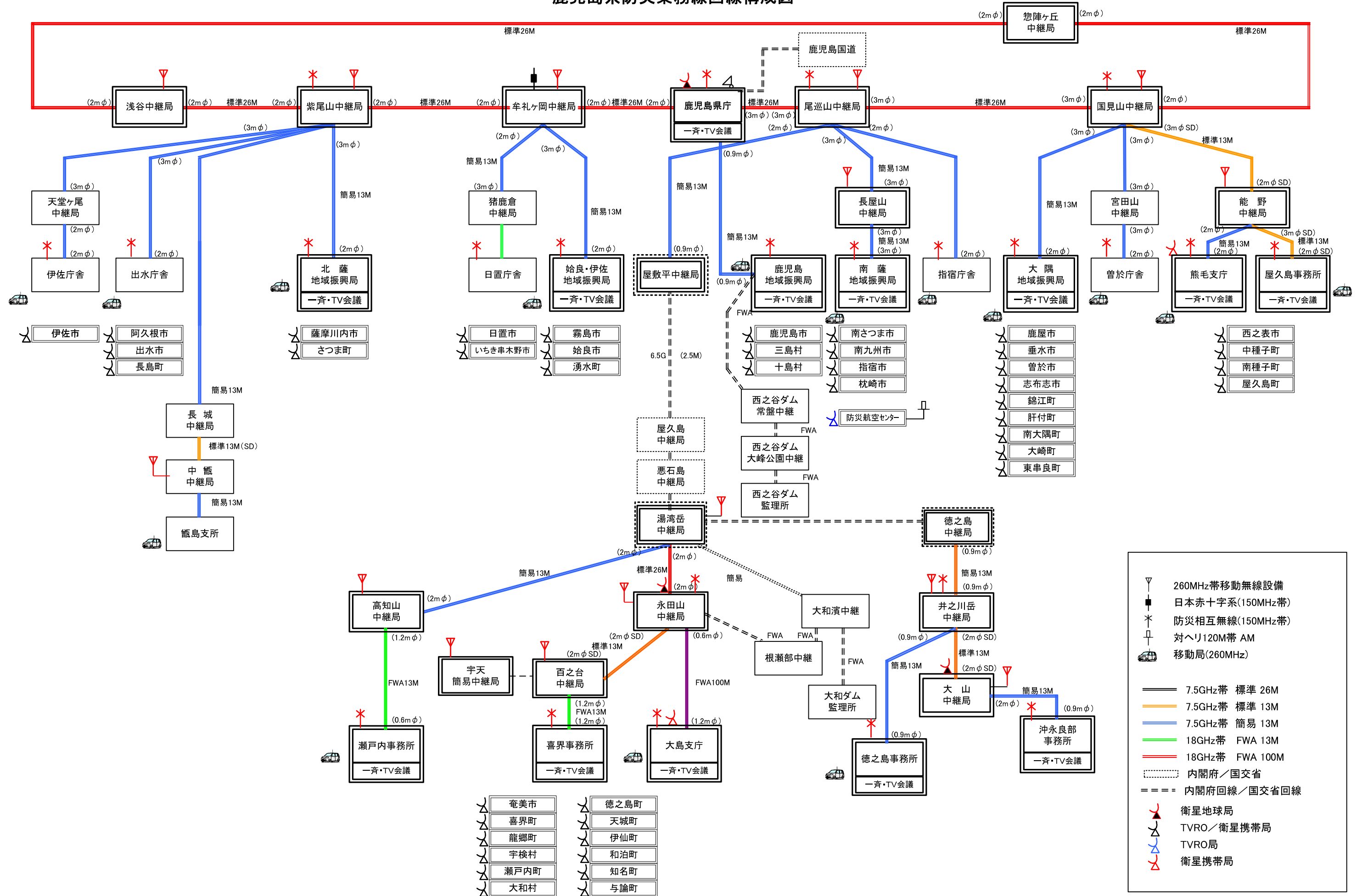
鹿児島県防災業務線回線構成図
