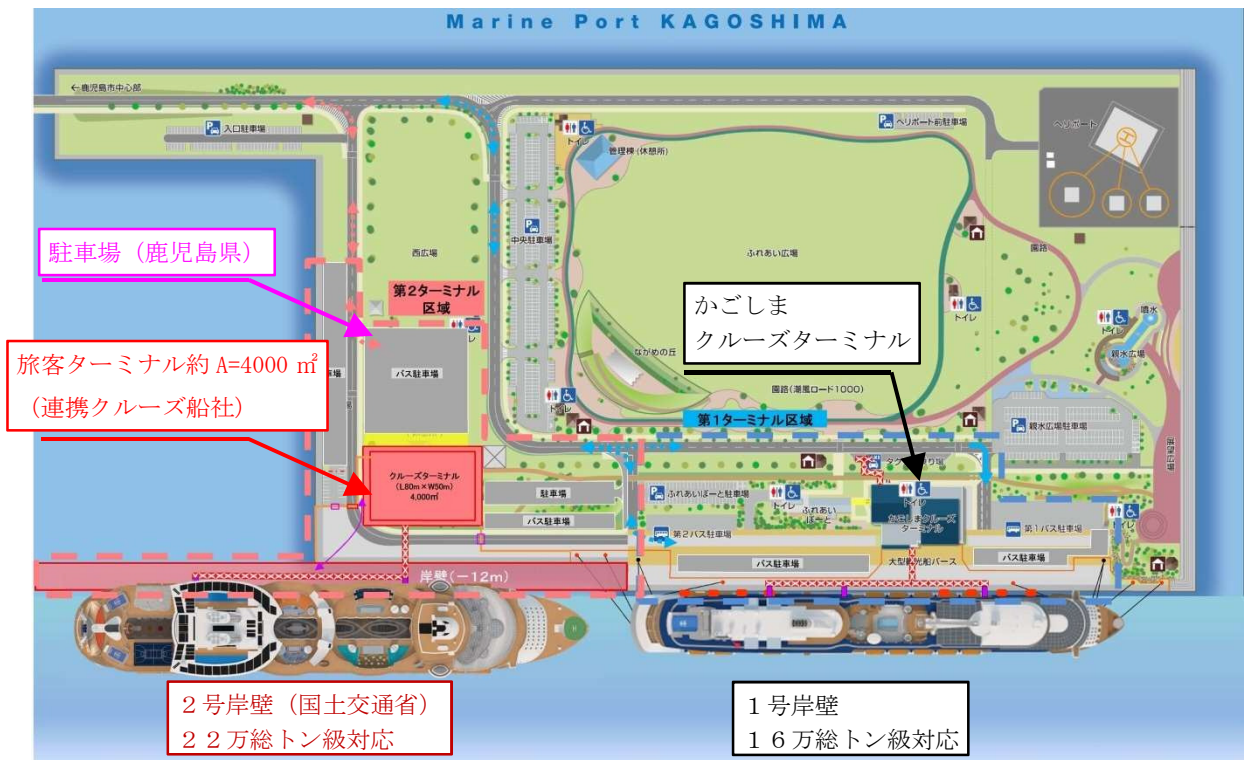
図-9 各施設の整備位置
