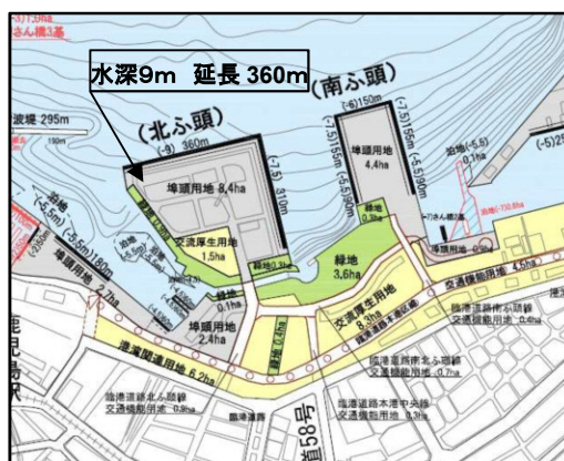
図-5 鹿児島港港湾計画〔本港区〕
