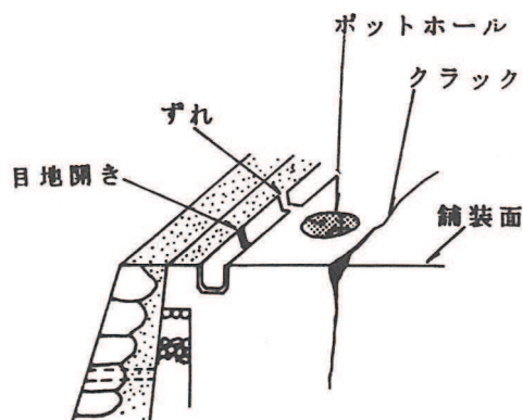
図 2 - 3 表面排水施設の被害状況例
