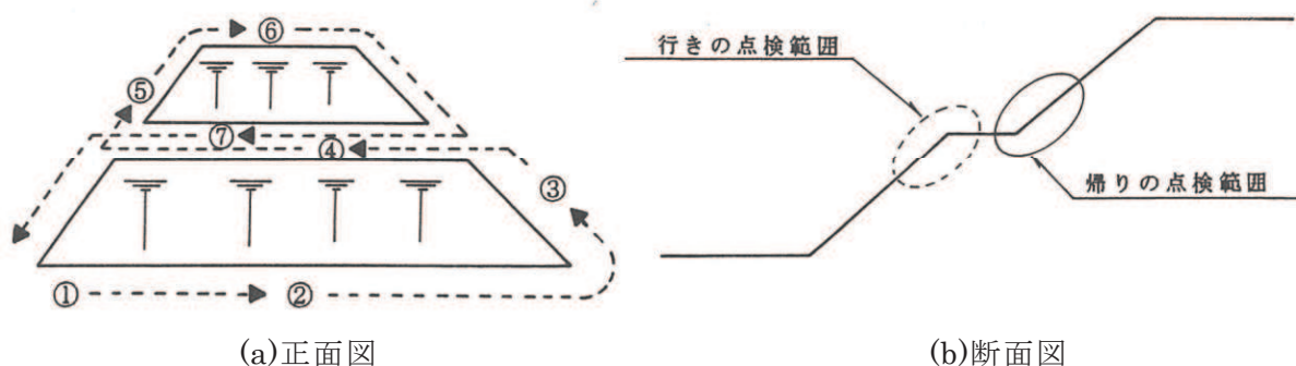
図 2 - 2 のり面の被害状況調査経路
