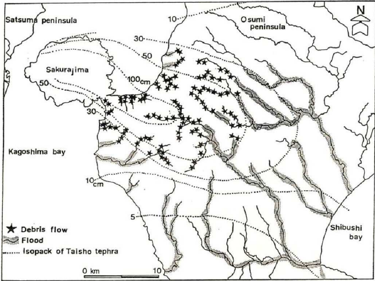
図 2-13 1914(大正3)年大噴火による軽石・火山灰の分布(金井, 1920 を改変)と土石流、洪水の発生
