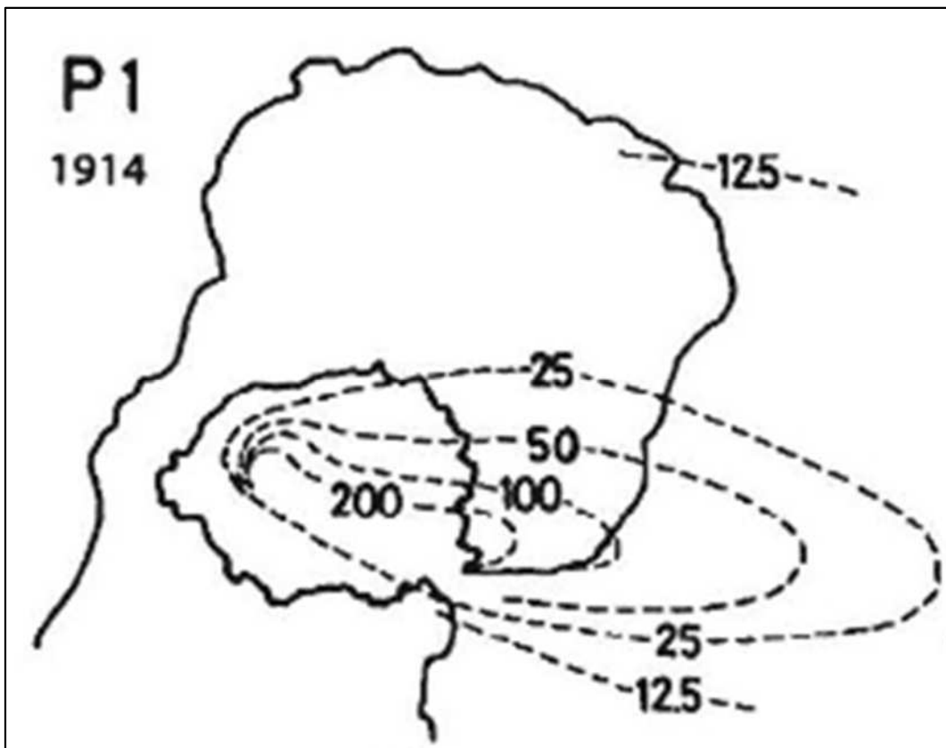
桜島火山地質図引用資料 (小林・溜池, 2002)
