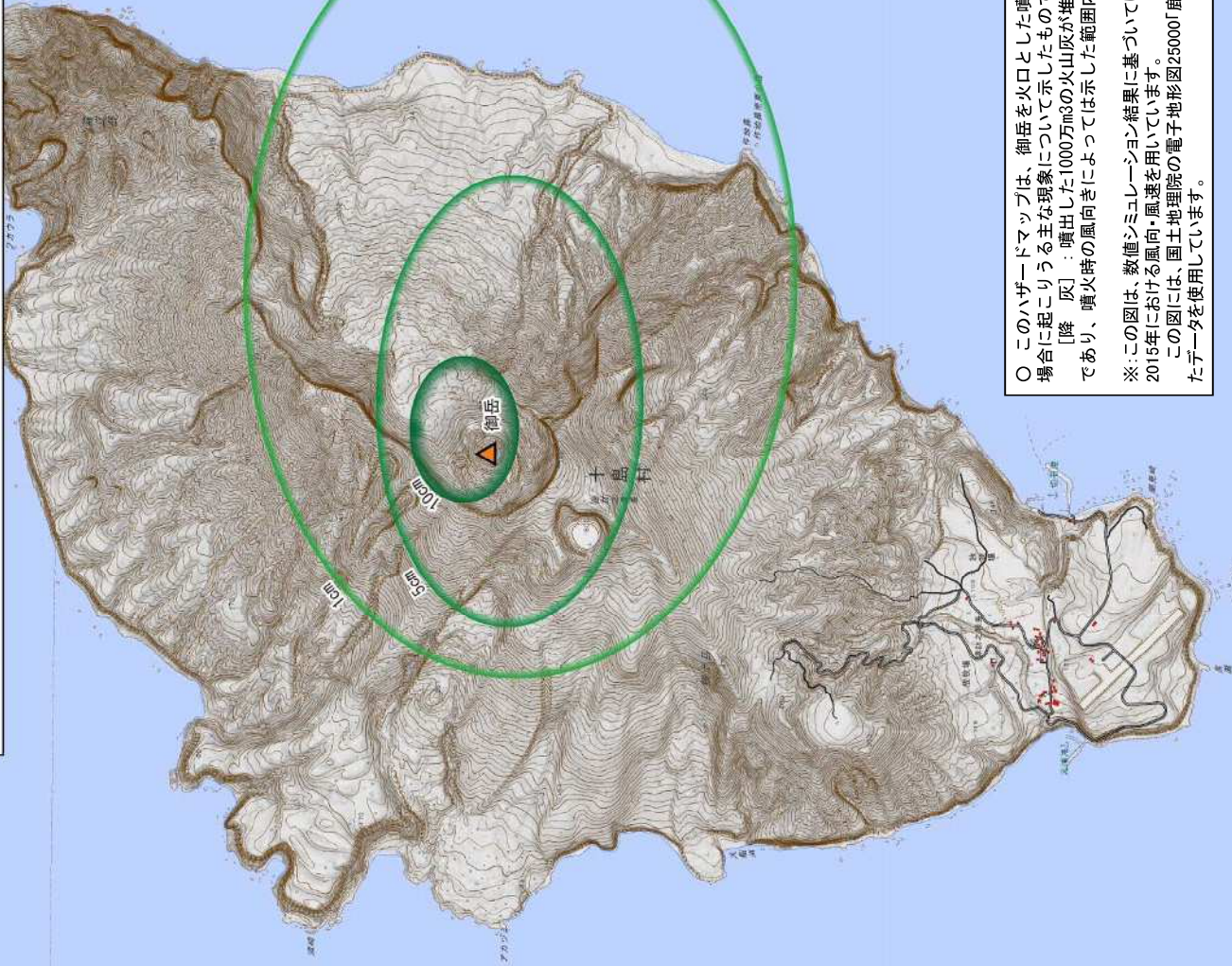
図5-5-3 諏訪之瀬島火山災害危険区域予測図 ⑬
