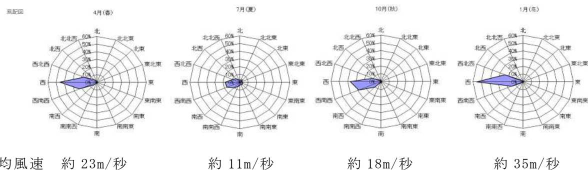
図3-1-2 季節ごとの風配図及び平均風速（上空5,500m付近）
