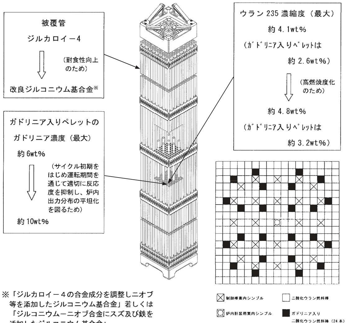
ガドリニア入り燃料棒配置図
