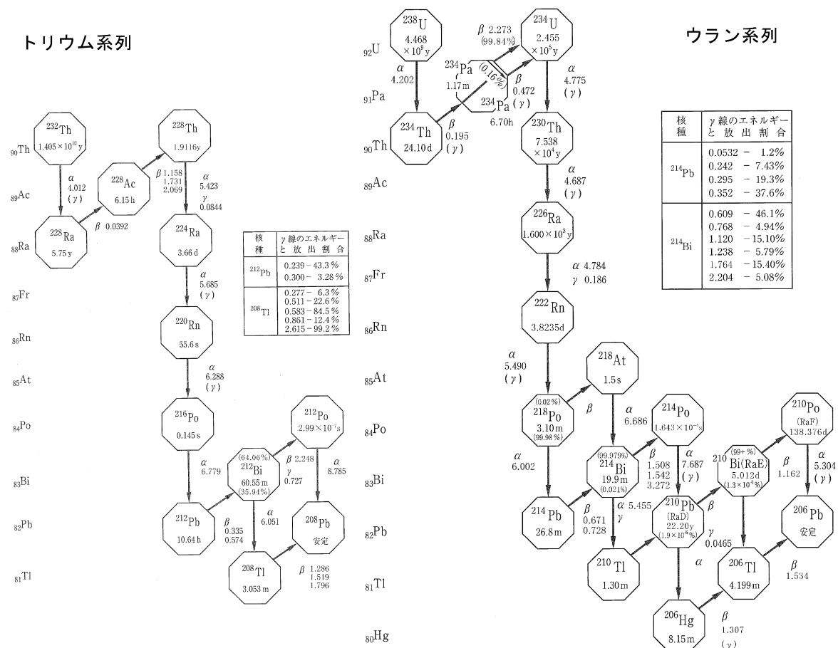
図1 トリウム系列とウラン系列
