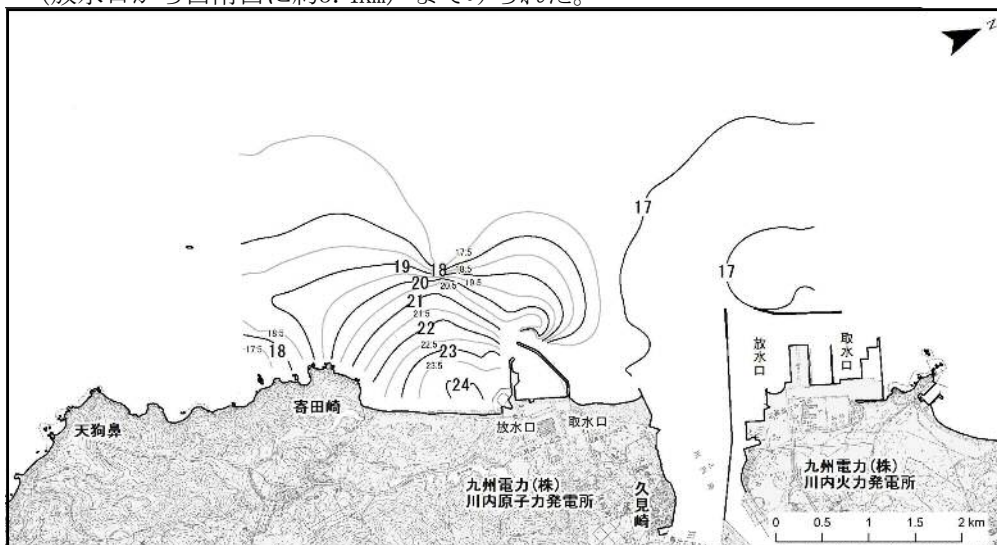
図6-1 表層（0.3m深）水温水平分布（上げ潮時） 単位：℃
