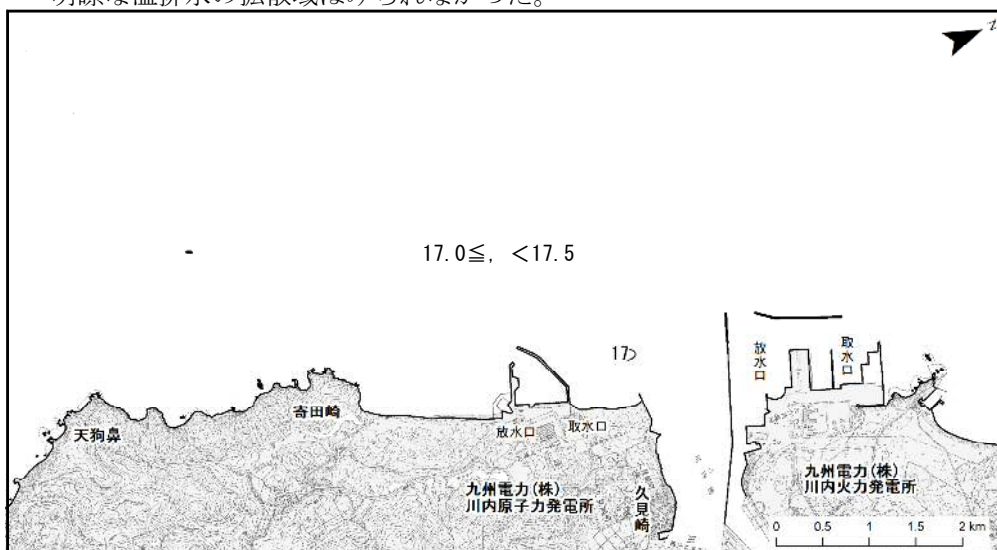
図6-4 3 m層水温水平分布（上げ潮時） 単位：℃
