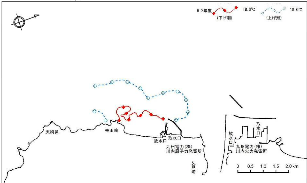
図8-10 令和2年度冬季表層(0.3m深)温排水拡散範囲
