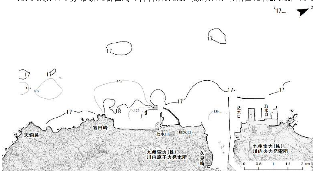
図5-2 1 m層水温水平分布（下げ潮時） 単位：℃
