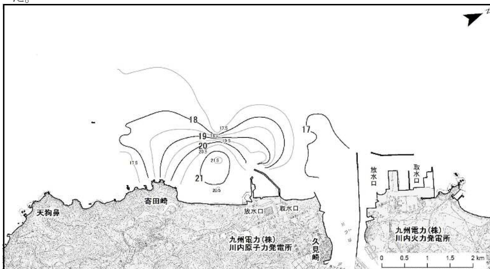
図6-2 1m層水温水平分布（上げ潮時） 単位：℃
