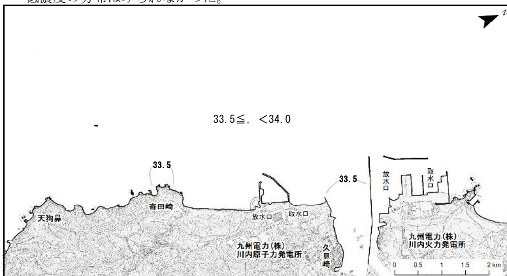
図7-1 表層（0.3m深）塩分水平分布（下げ潮時）
