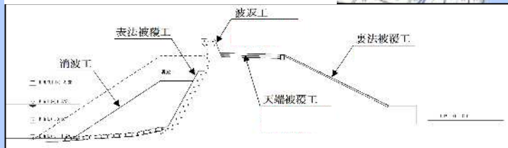
一定区間No.2 海岸堤防断面図
