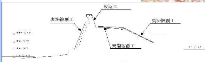
一定区間No.1 海岸堤防断面図
