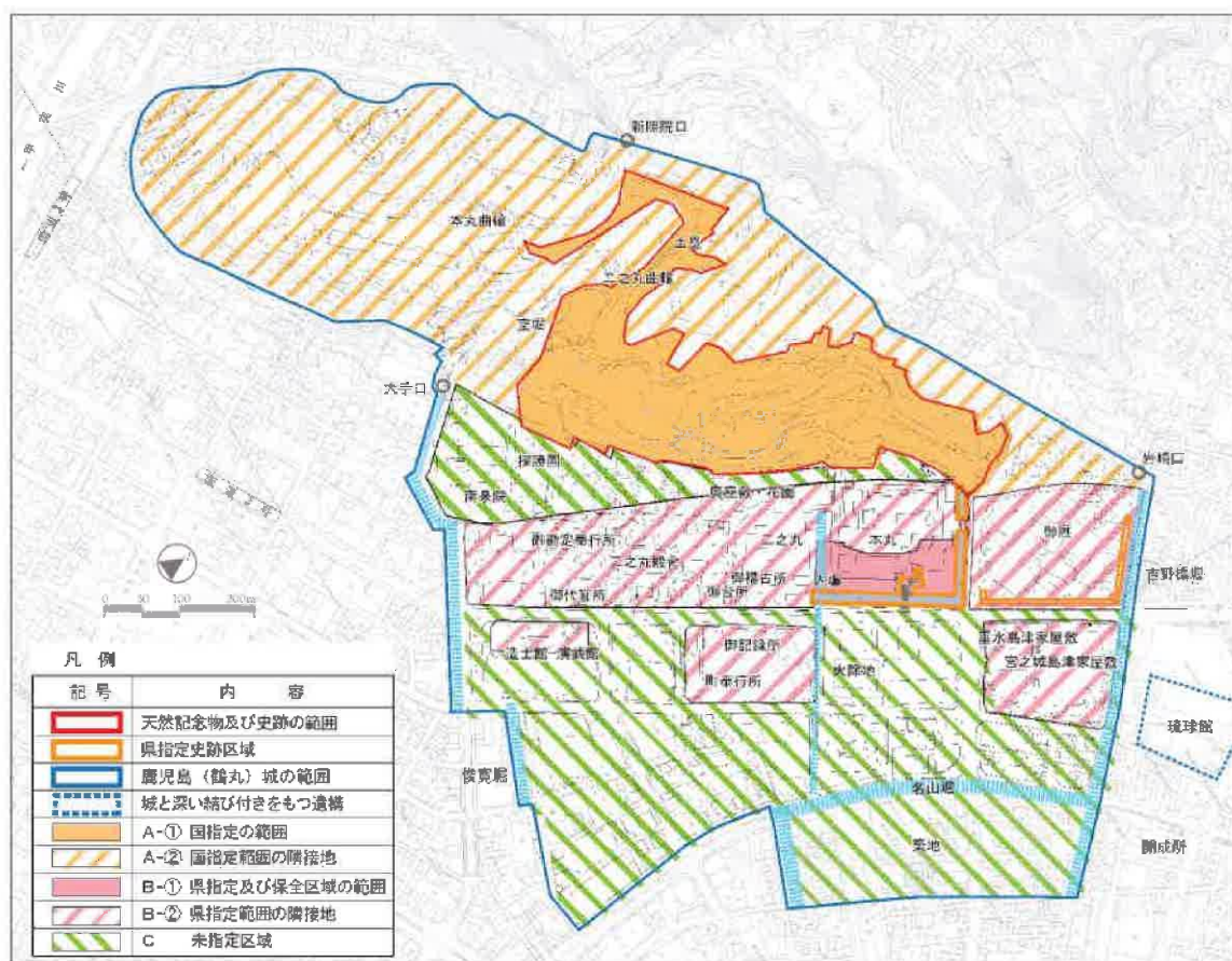
図 1-4 地区区分図
