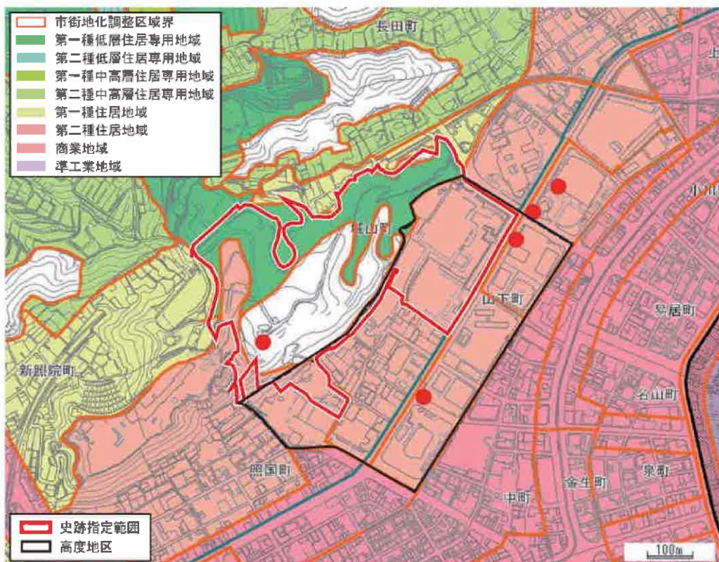
図 1-9 用途地域図
