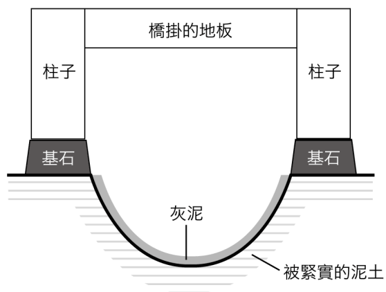
▲橋掛的下層結構
