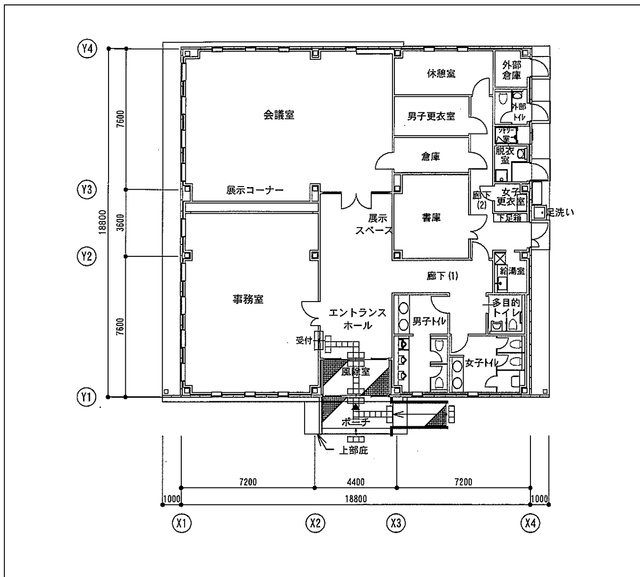
図 34 管理棟の平面図
