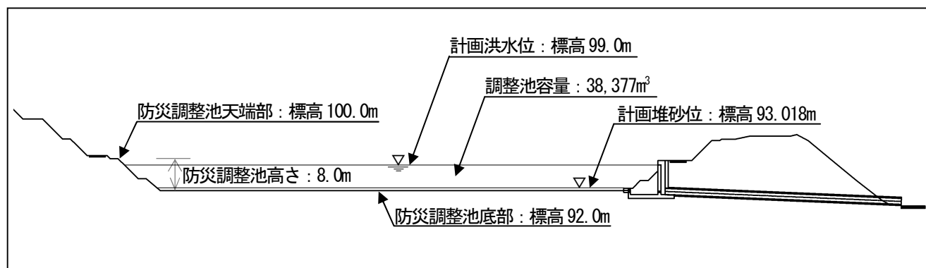
図 44 防災調整池の断面図 (A-A' 断面)
