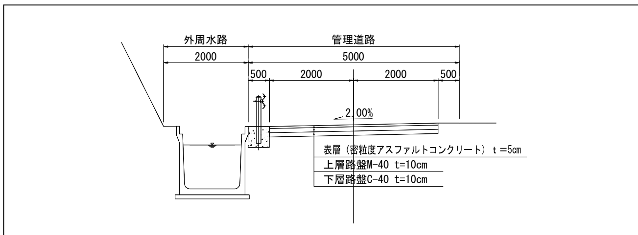
図 40 道路施設（管理道路）の標準構造図
