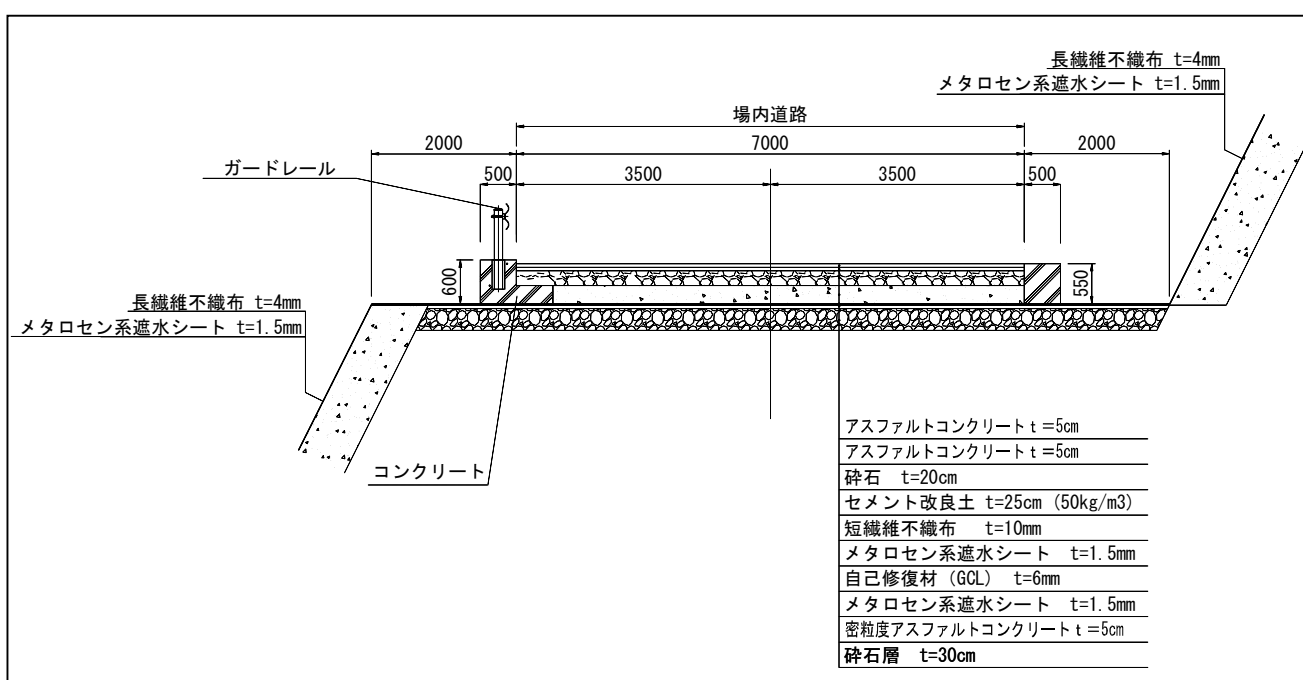
図 42 道路施設（場内道路）の標準構造図
