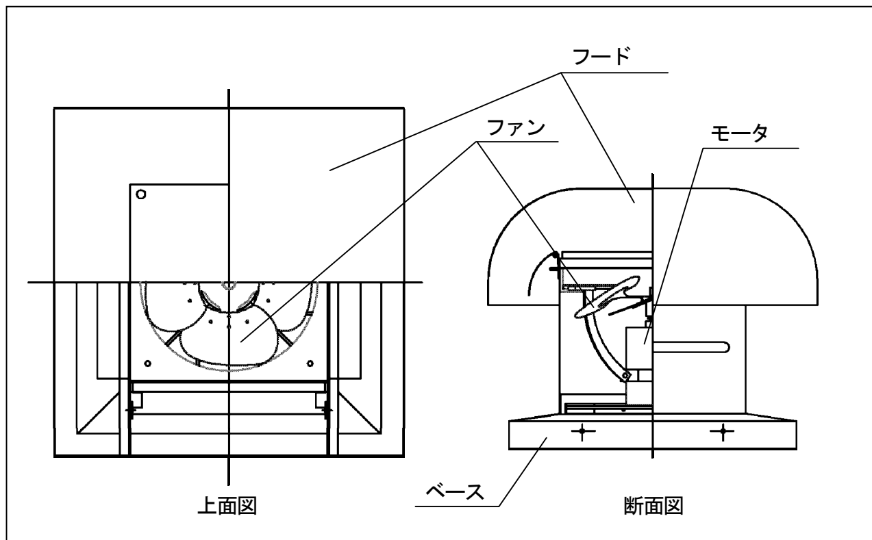
図 32 排気装置の一般構造図
