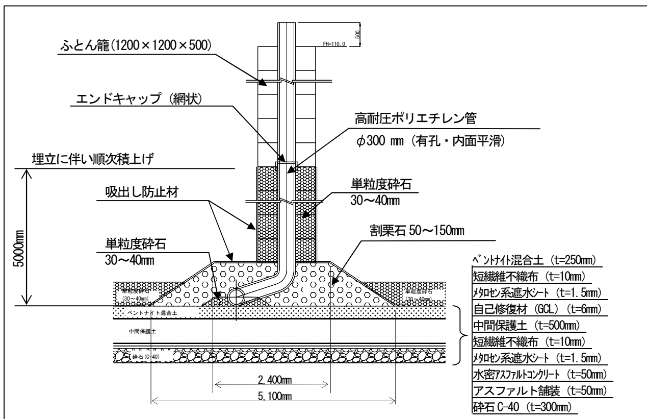
図 29 ガス処理施設（縦型）の標準構造図
