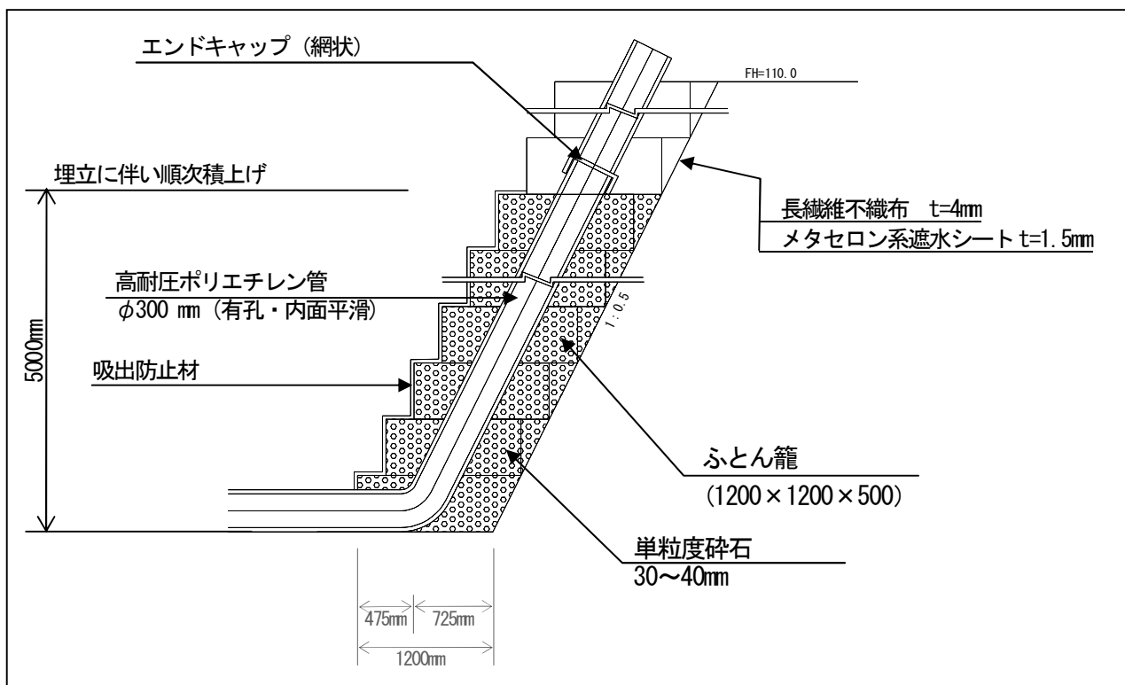
図 30 ガス処理施設（法面）の標準構造図
