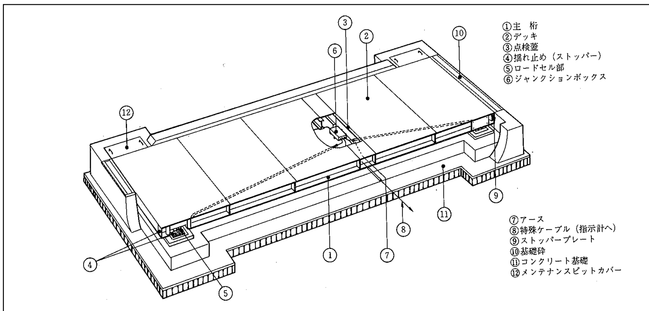
図 36 トラックスケール（ロードセル方式）の一般構造図
