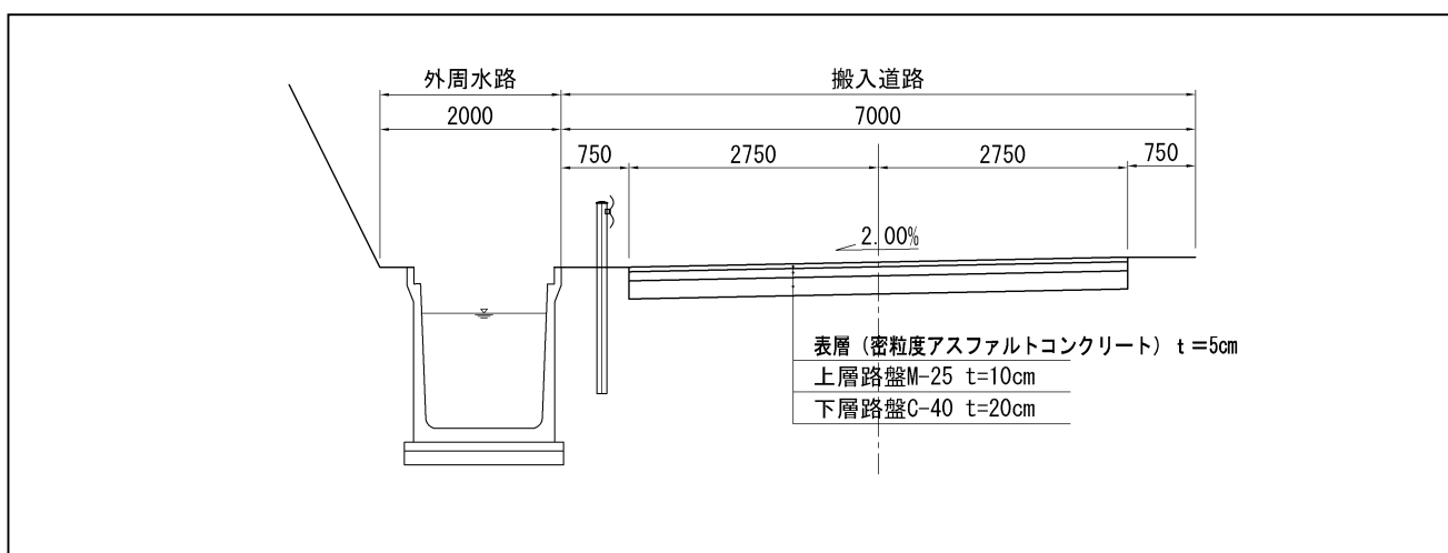
図 41 道路施設（搬入道路）の標準構造図
