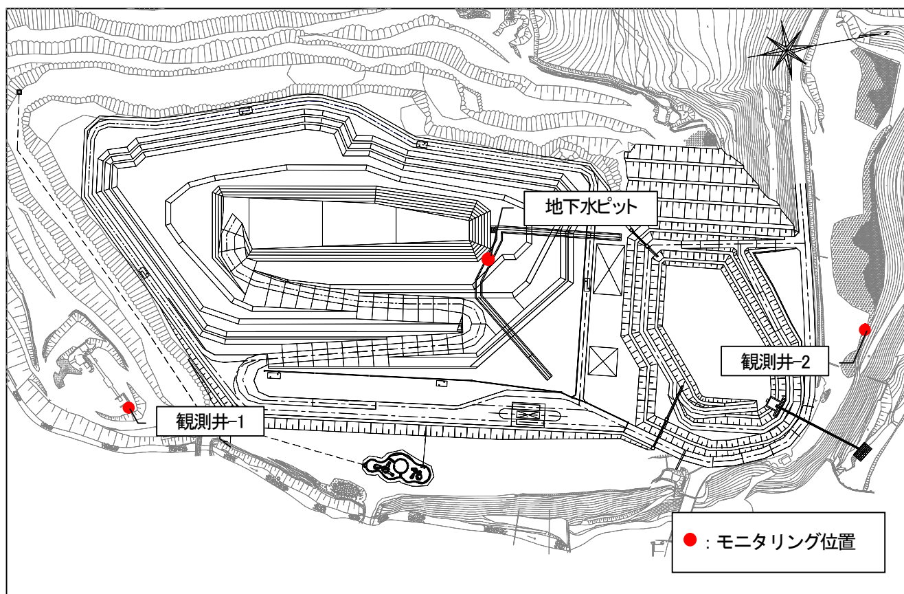
図 38 環境モニタリング施設の平面図
