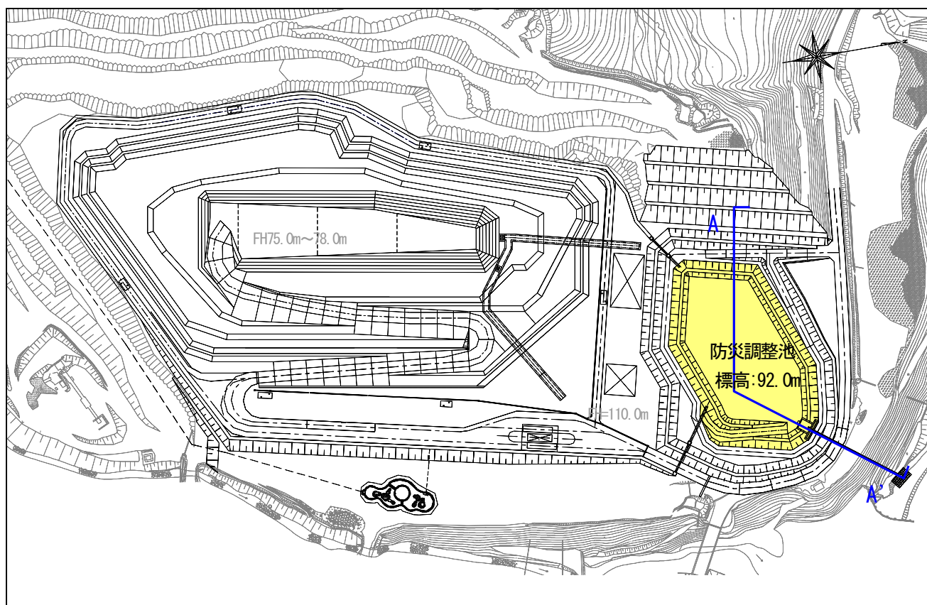
図 43 防災調整池の平面図
