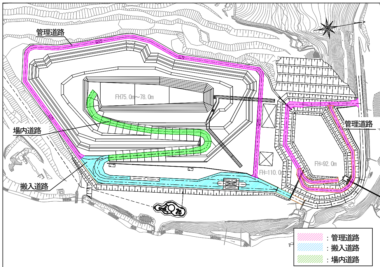
図 39 道路施設の平面図
