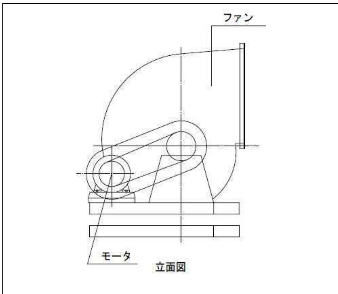
図 31 給気装置の一般構造図
