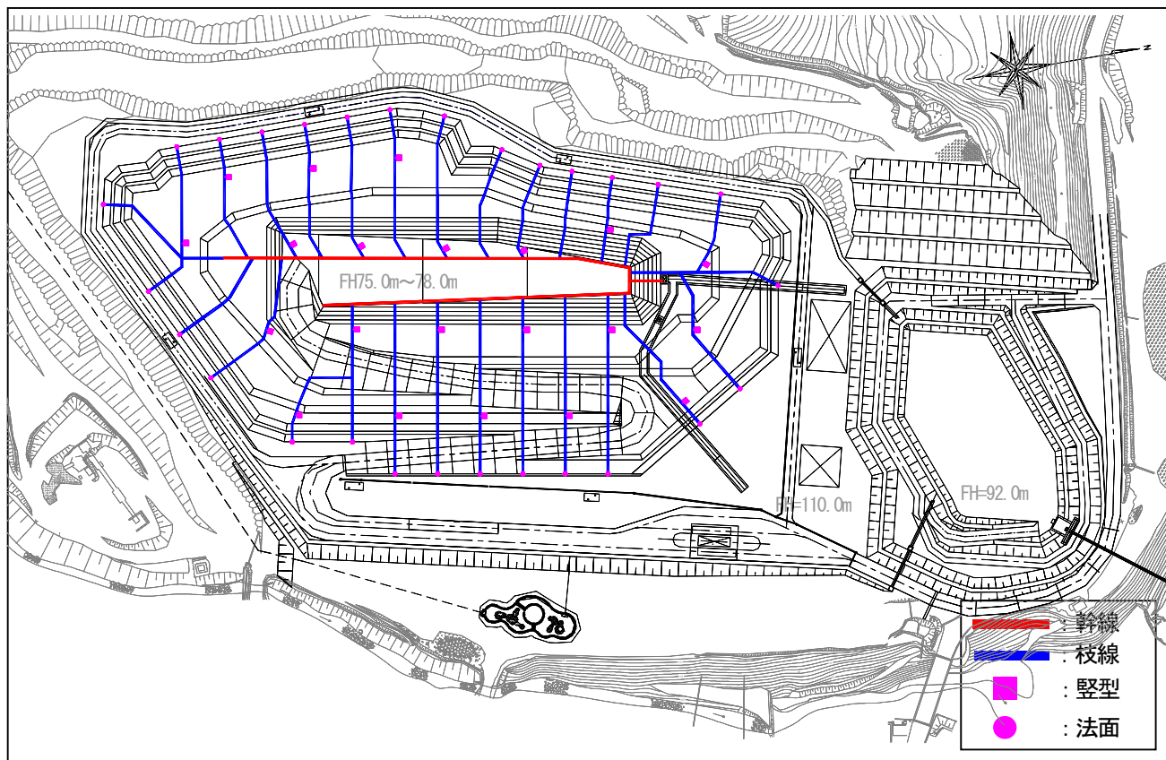
図 28 ガス処理施設平面図
