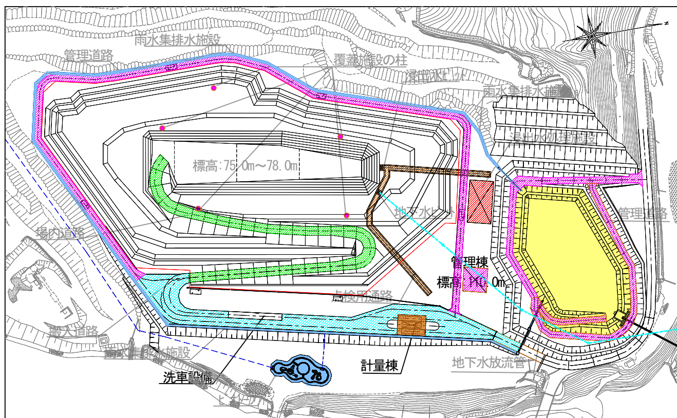
図 33 管理施設の配置図
