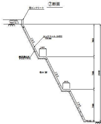
一般構造図(背面岩盤)
