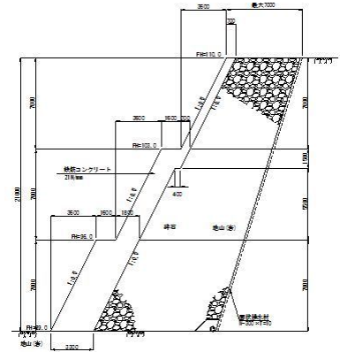
一般構造図(背面砕石)
