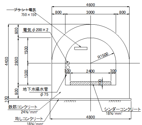
標準断面図
