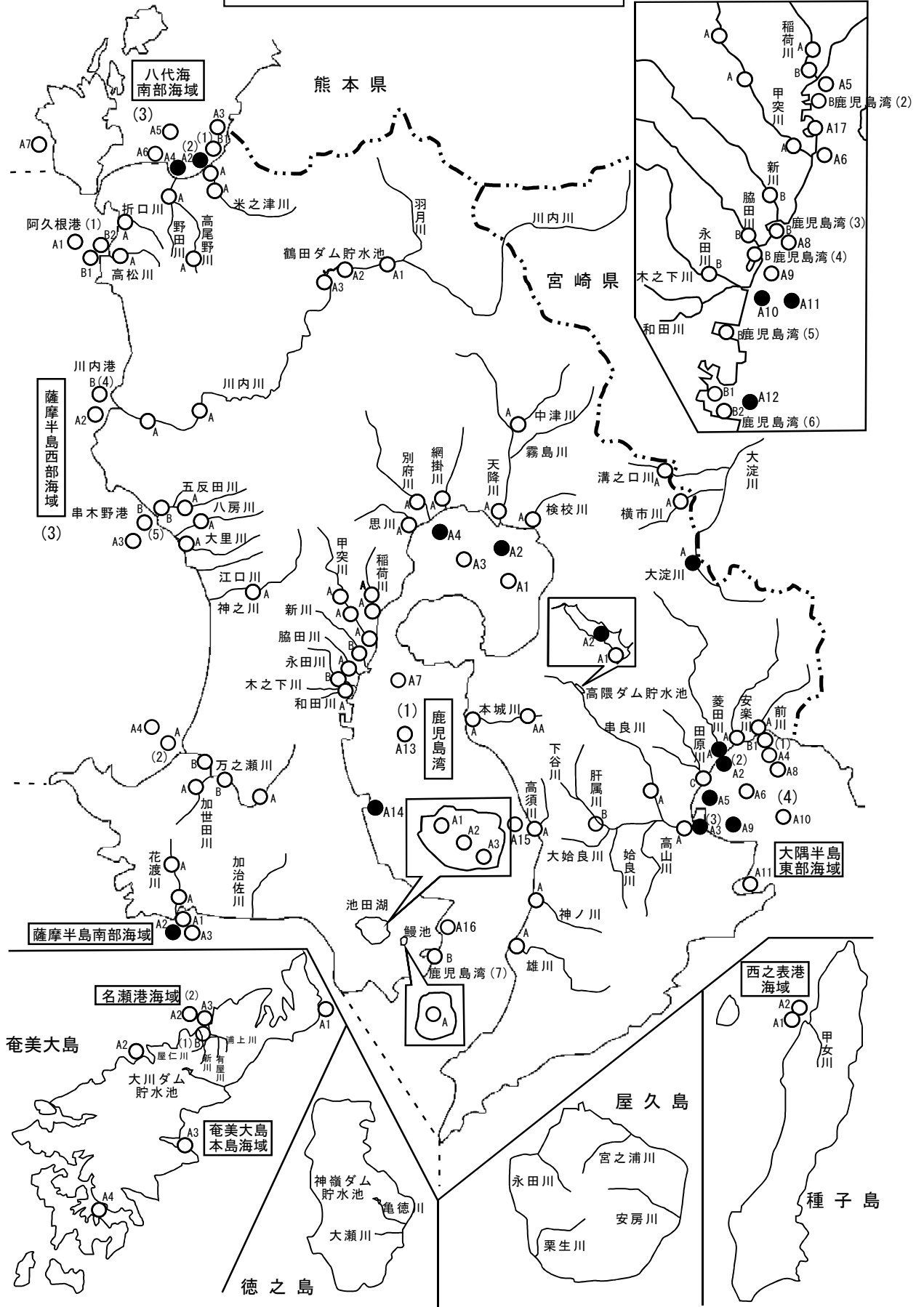
図-3 令和4年度環境基準 (BOD又はCOD) 達成状況図
