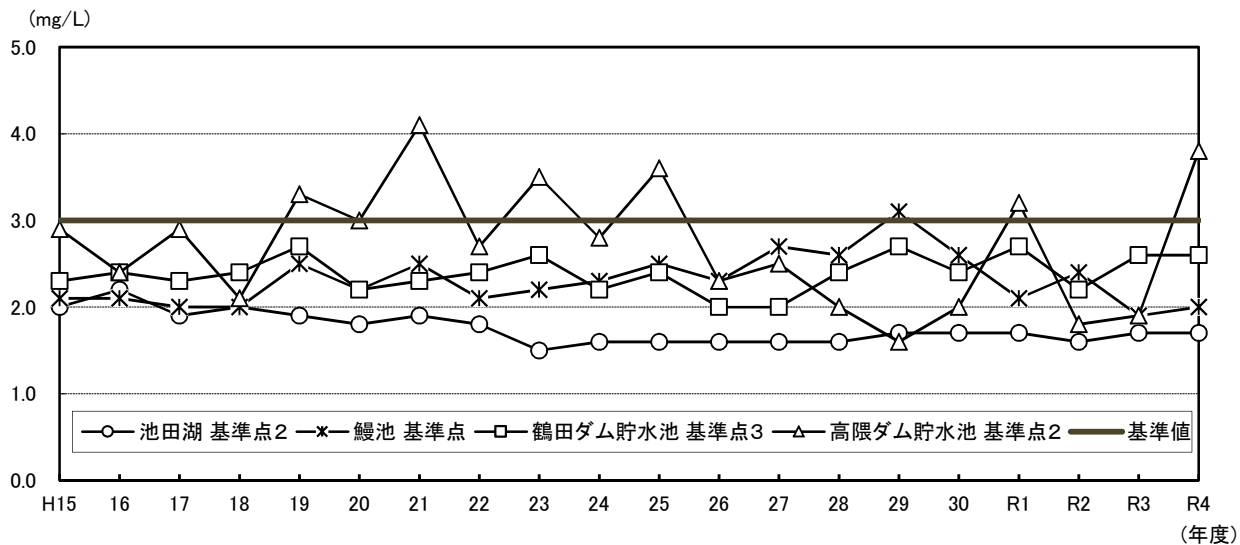
(2) COD75%値の経年変化(基準点の最大値と最小値)
