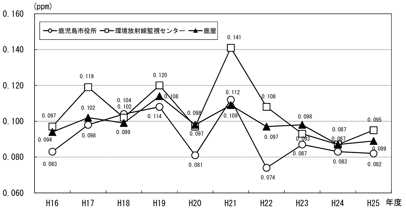
図4 光化学オキシダント (Ox) の昼間の1時間値の最高値の推移
