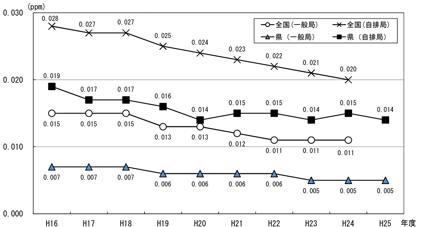
図3 二酸化窒素（NO 2 ）の年平均値の推移
