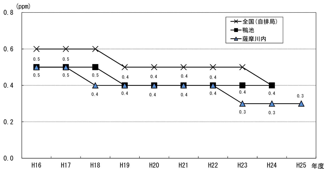
図5 一酸化炭素（CO）の年平均値の推移
