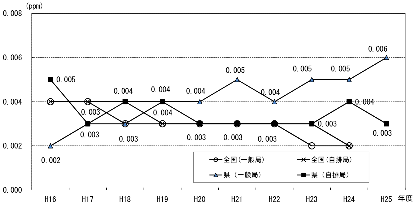
図 1 二酸化硫黄 (SO 2 ) の年平均値の推移
