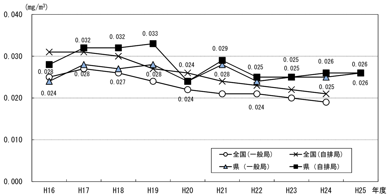
図2 浮遊粒子状物質（SPM）の年平均値の推移
