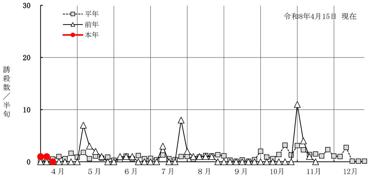
フェロモントラップによるオオタバコガの誘殺状況 (南さつま市金峰町)
