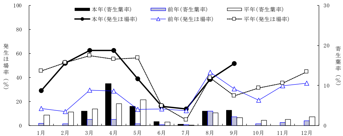
図1 カンザワハダニの発生ほ場率と寄生葉率の推移
