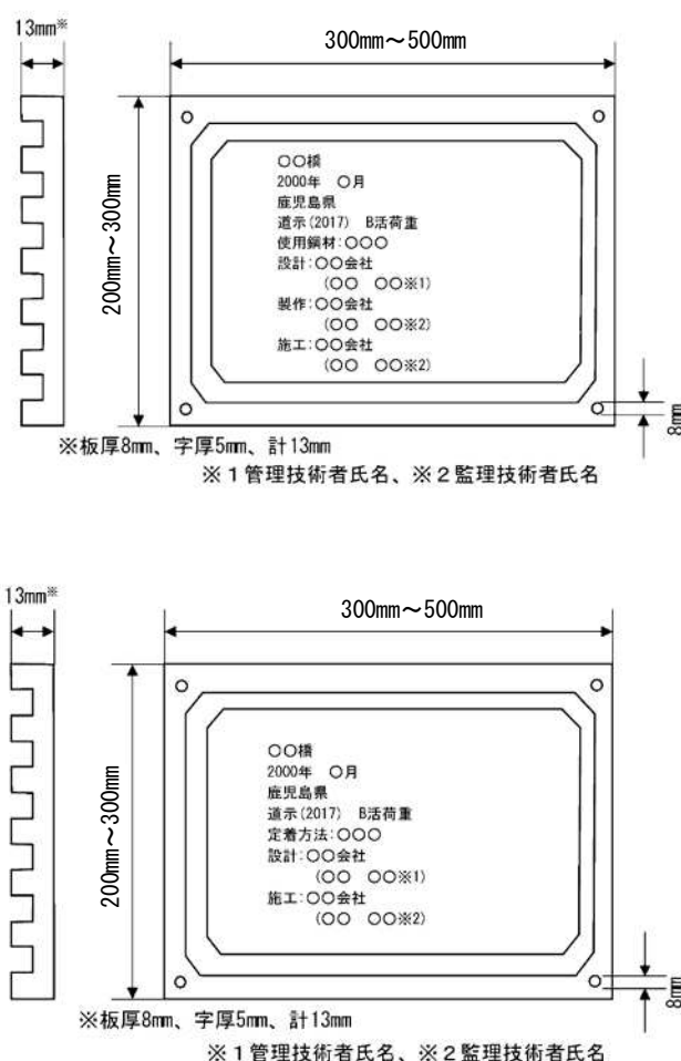
図3-2-2 銘板の寸法及び記載事項
