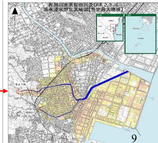
木之下川の浸水想定区域図（一部抜粋）
