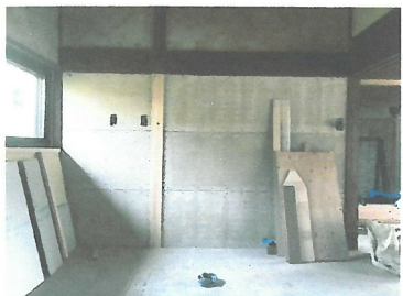
●古い構造体は、古民家再生に利用される A／「荒壁パネル」 B／「筋交い」で補強する
