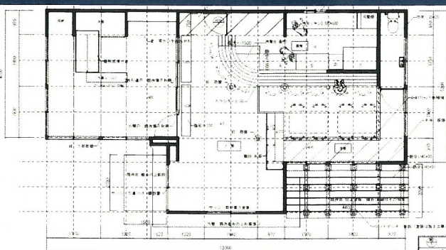
【設計図】
