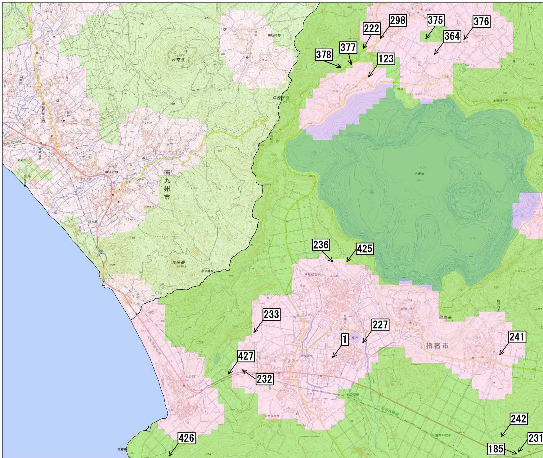
宅地造成等工事規制区域 及び特定盛土等規制区域図 (指宿市)
