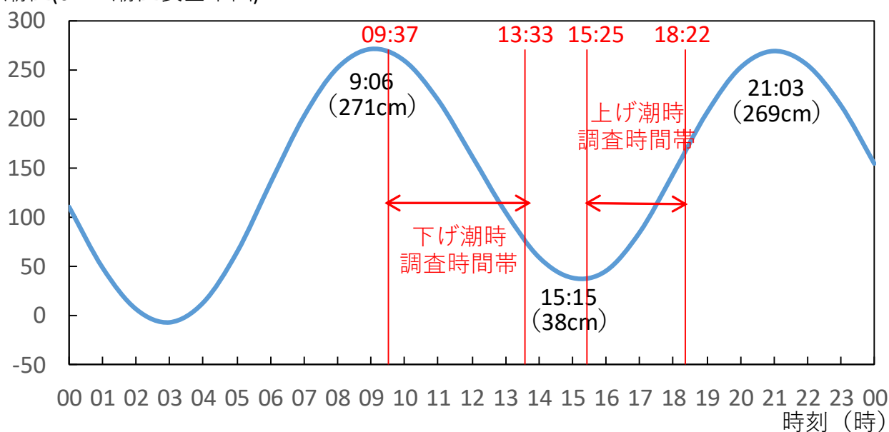
図3 水温・塩分水平分布調査日(令和4年3月4日)の潮汐(阿久根験潮場)と調査時間
