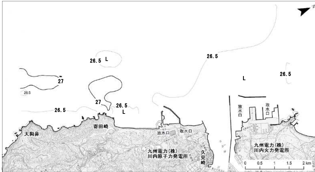
図9-3 2m層水温水平分布（下げ潮時） 単位：℃
