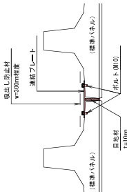
ハネル目地部
