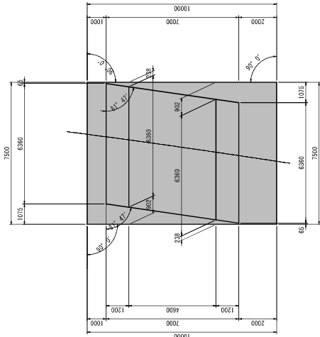
底版平面図 (5 - 5)
