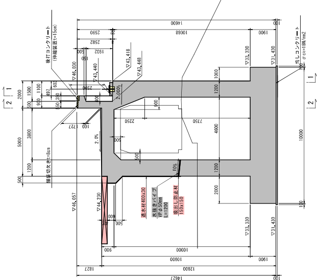
断面図 (3 - 3)
