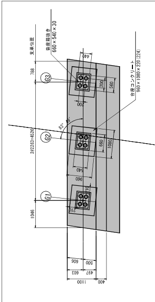
平面図 S=1:50
