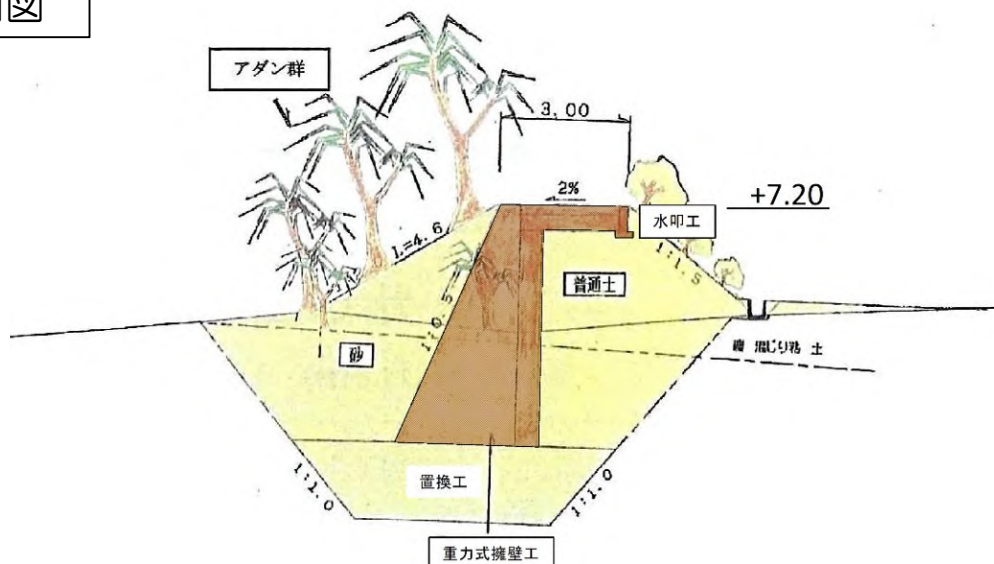
断面図
