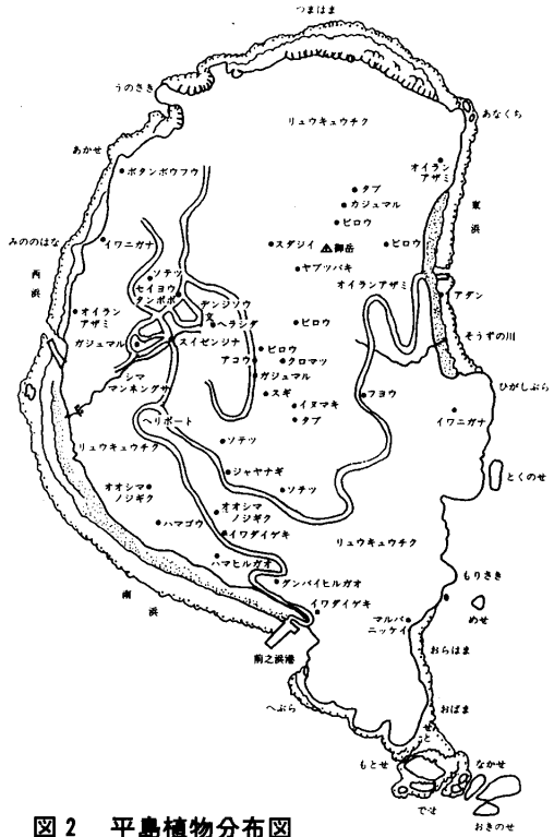
図2 平島植物分布図 平島小岡村清教諭(原図)に追訂
