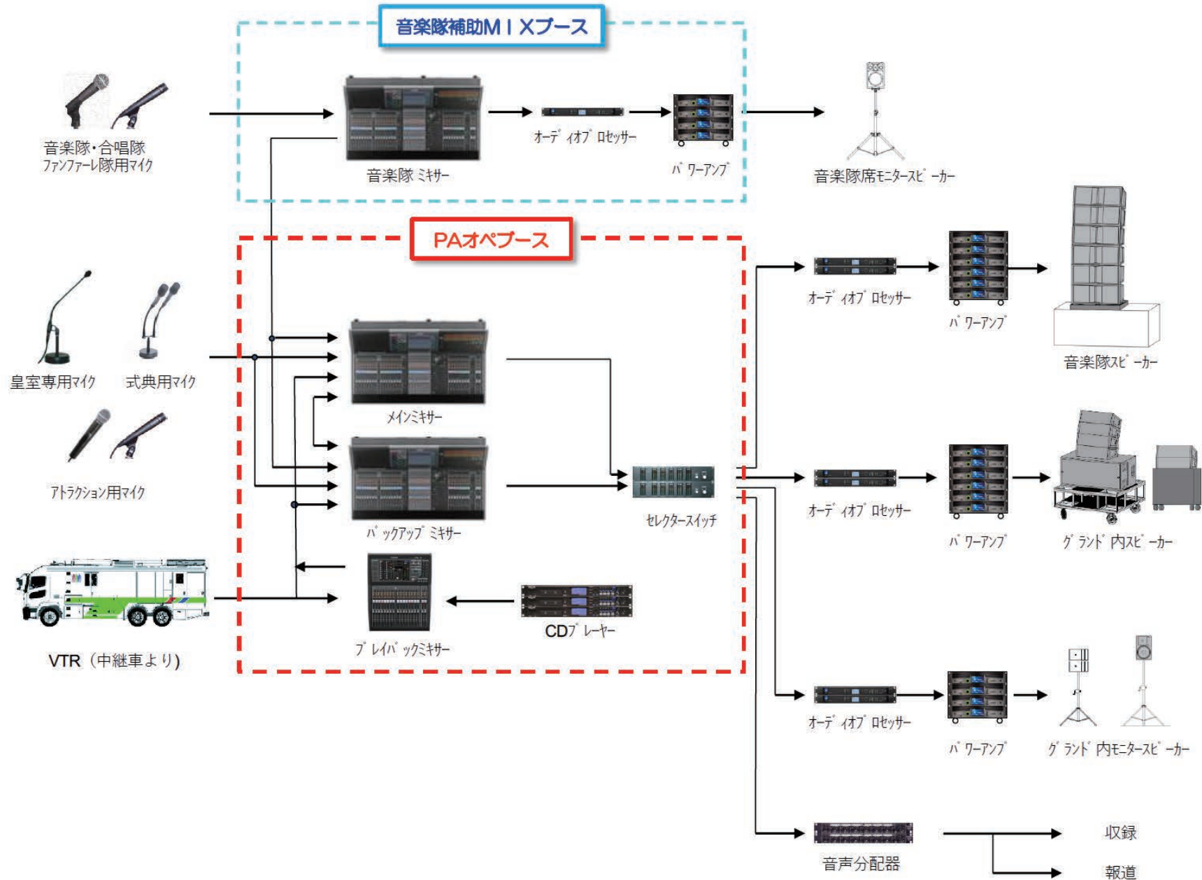
(2) 音響システム図
